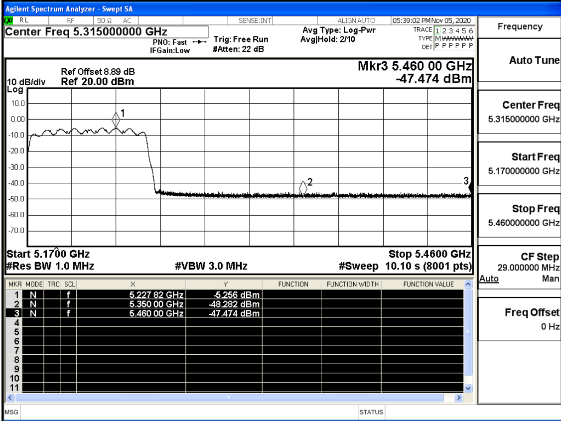
IEEE 802.11ac80 / Channel 42/ 5210MHz / Peak
