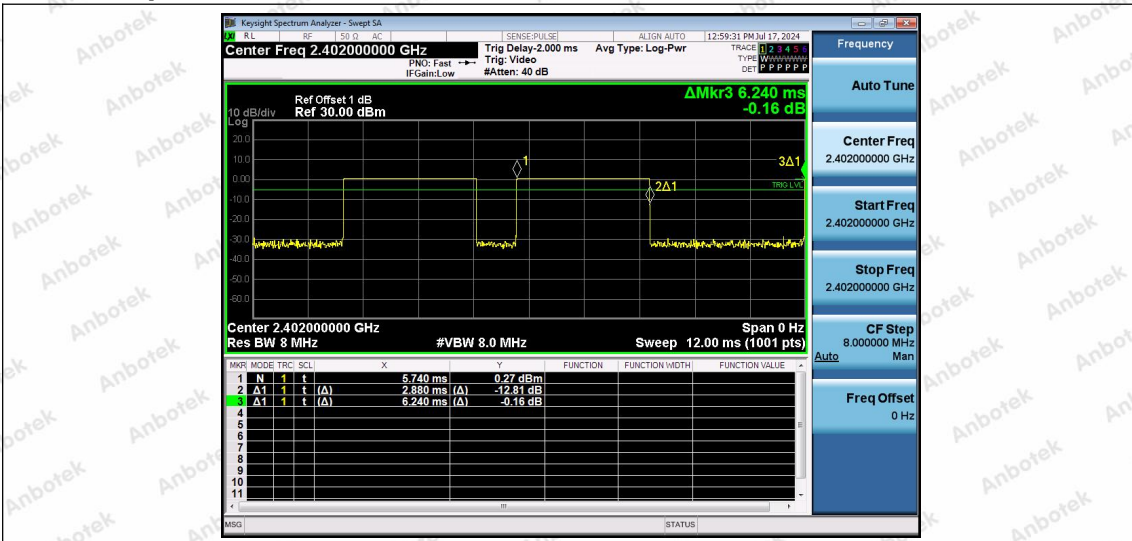
NTNV-2.4G-Ant1-2402
