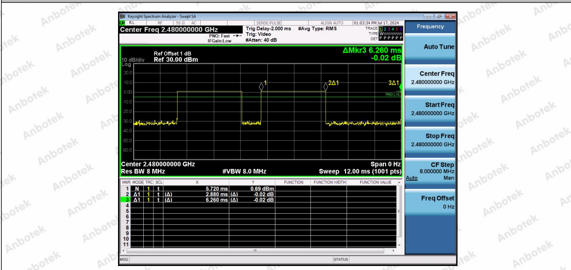
NTNV-2.4G-Ant1-2480
