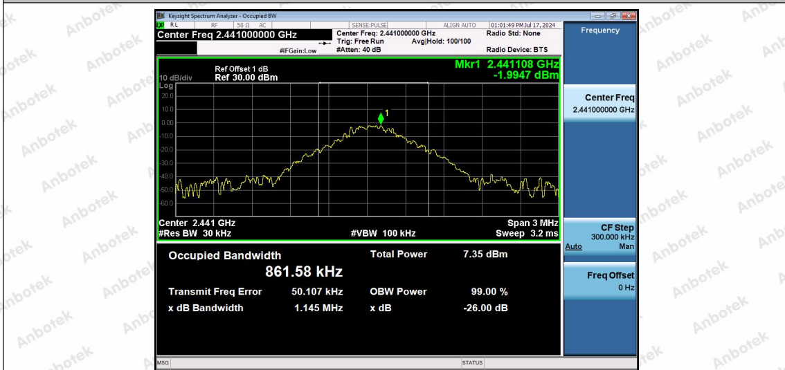
2.4G-Ant1-2441
