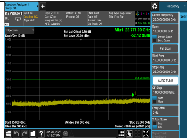
802.11n(HT20),2462MHz,Ant0,Plot 6,15000MHz~25000MHz
