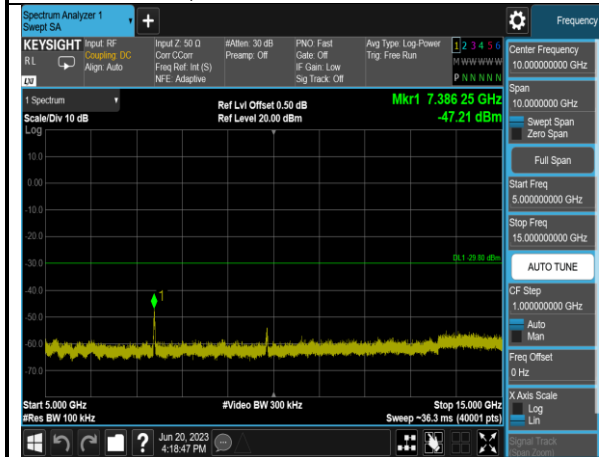
802.11n(HT20),2462MHz,Ant0,Plot 5,5000MHz~15000MHz
