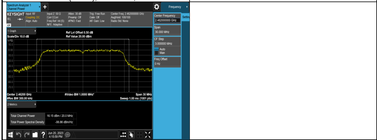
802.11n(HT20),2462MHz,Ant0
