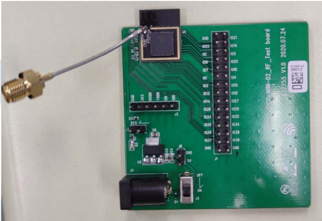
a: EUT
