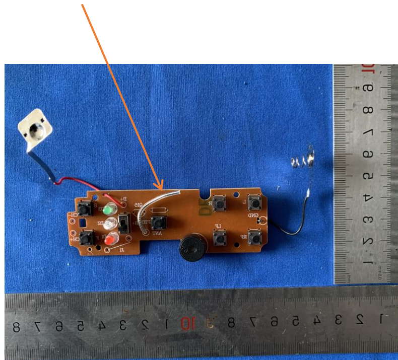
Antenna
