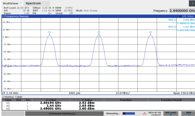
BLE 2 Mbps
