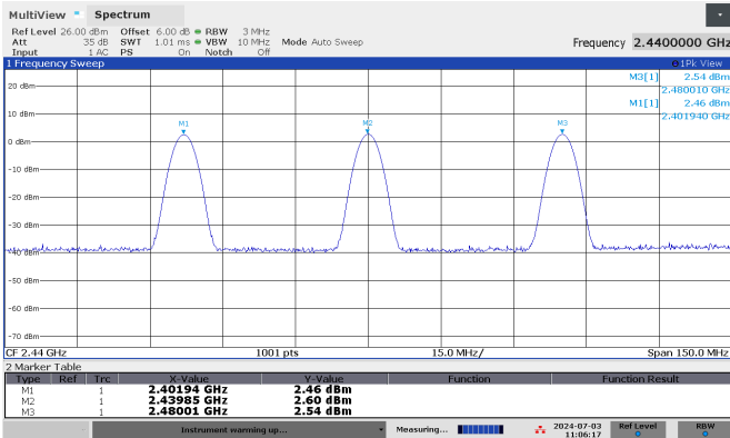
BLE 2 Mbps
