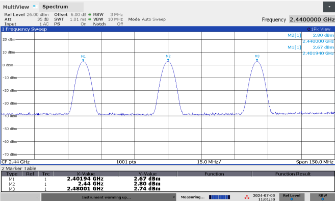
BLE 1 Mbps
