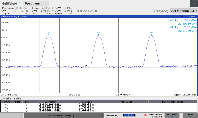
BLE 1 Mbps
