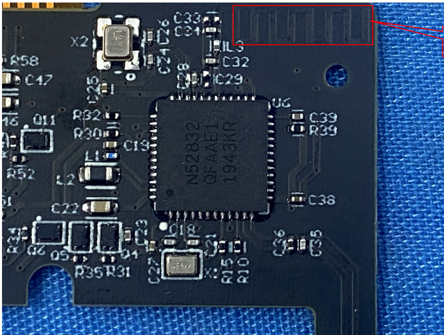
BLE Antenna
