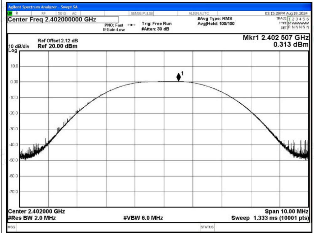
Power NVNT BLE 2M 2402MHz Ant1
