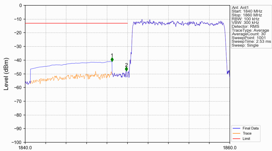
Band2_10MHz_16QAM_LCH_1855MHz_RB_50_0_NTNV
