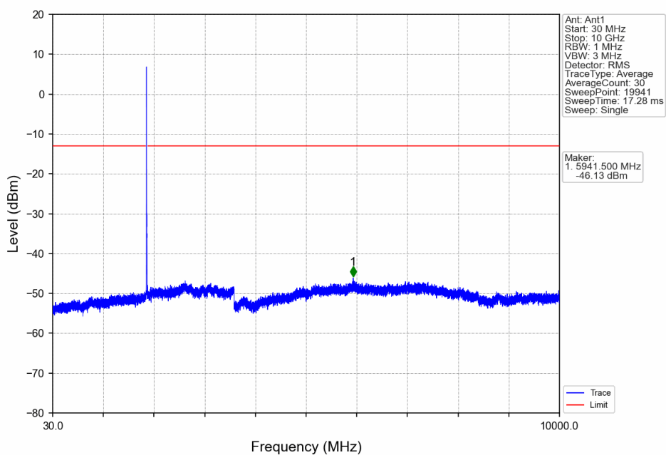
Band2_10MHz_QPSK_MCH_1880MHz_RB_1_0_NTNV
