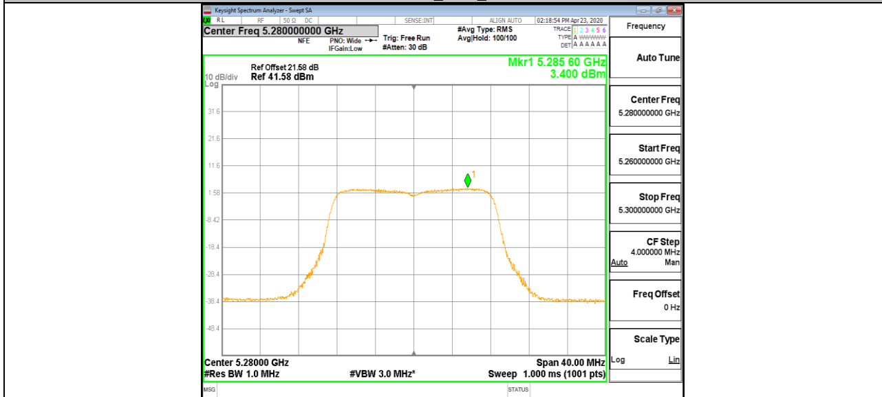
11A-CDD_Ant2_5280
