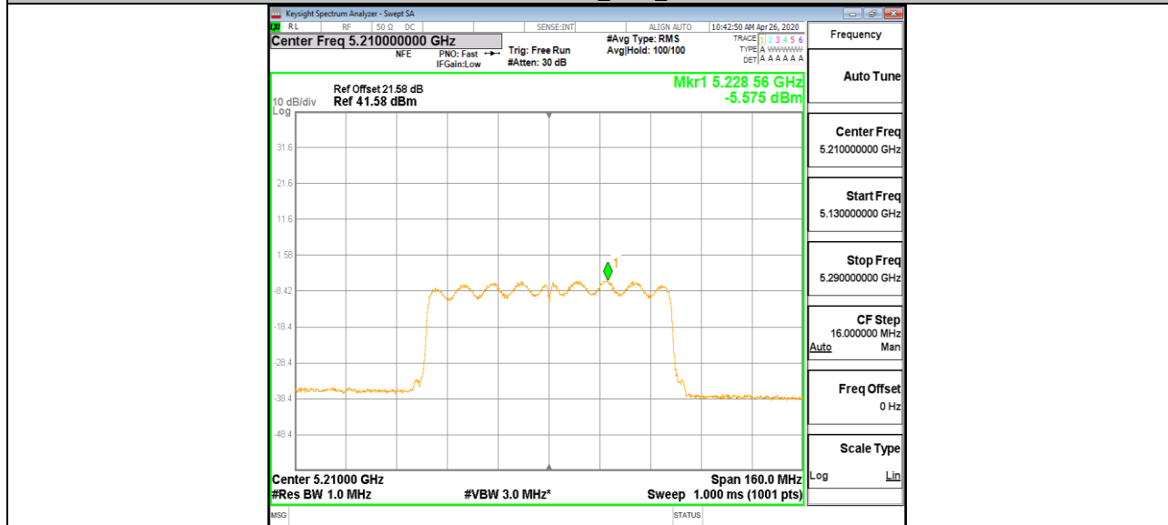
11AC80MIMO_Ant2_5210
