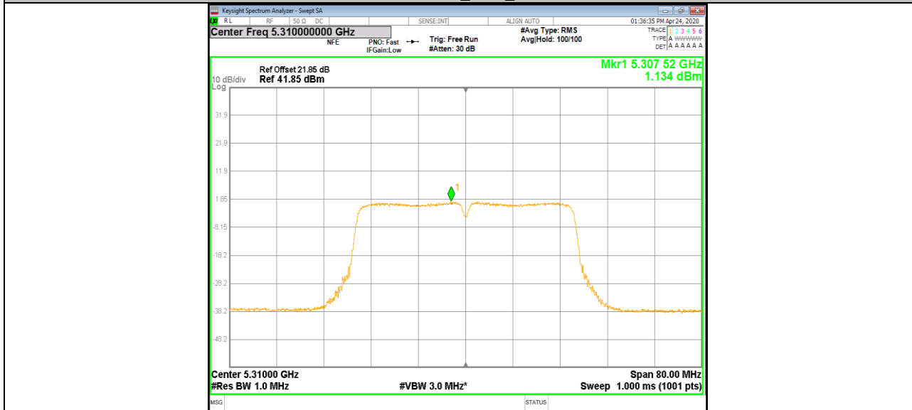
11N40MIMO_Ant2_5310
