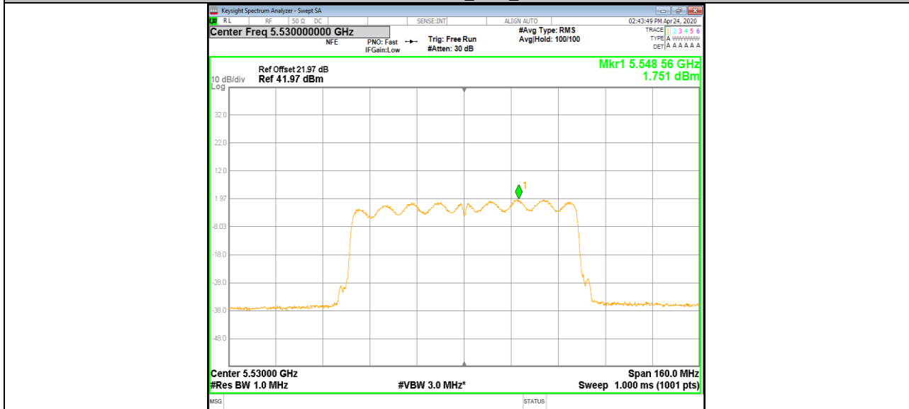
11AC80MIMO_Ant2_5530
