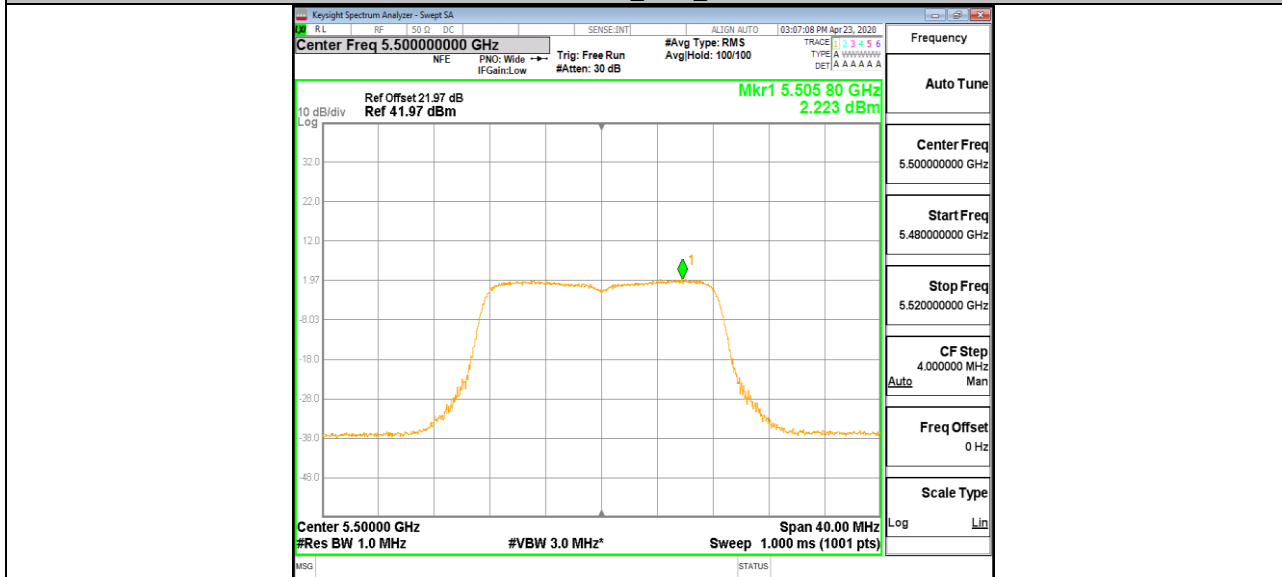
11A-CDD_Ant2_5500
