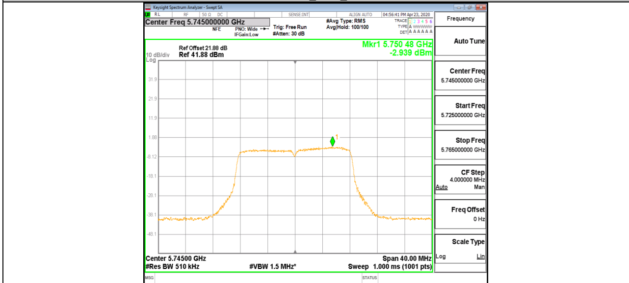
11A-CDD_Ant2_5745
