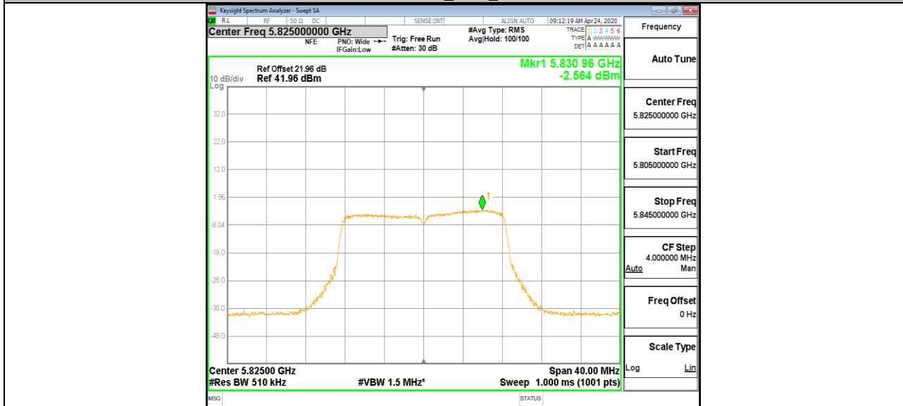
11A-CDD_Ant2_5825
