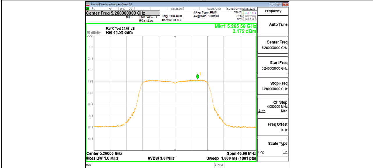
11A-CDD_Ant2_5260
