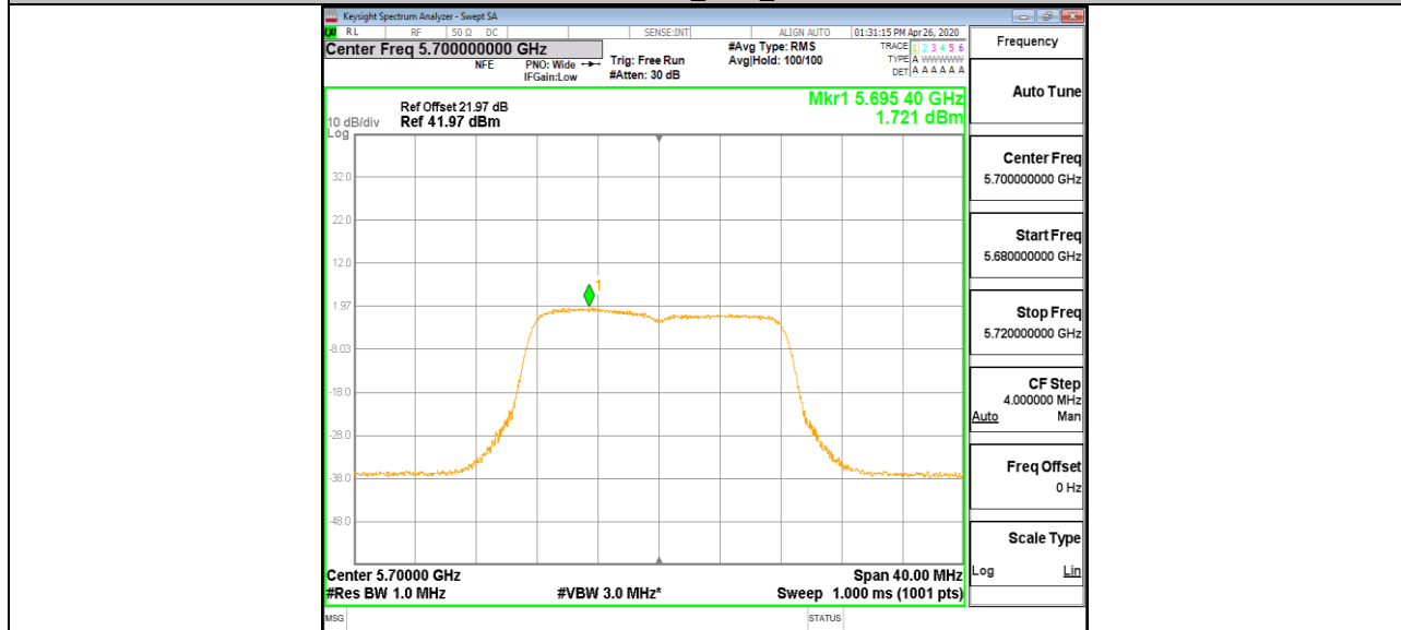
11A-CDD_Ant2_5700
