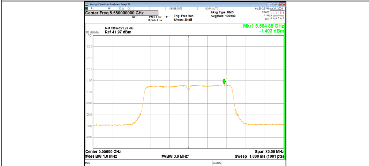
11N40MIMO_Ant2_5550
