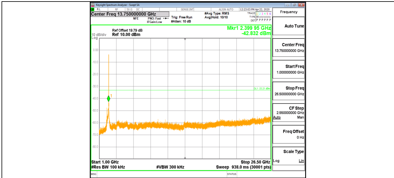
11N40MIMO_Ant2_2422_0~Reference
