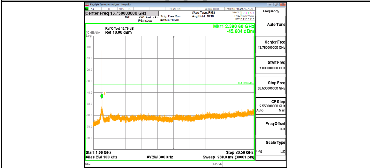
11N40MIMO_Ant1_2437_0~Reference
