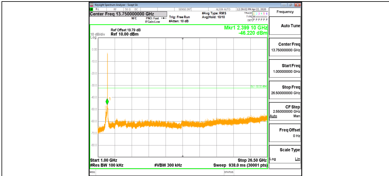
11N40MIMO_Ant2_2437_0~Reference
