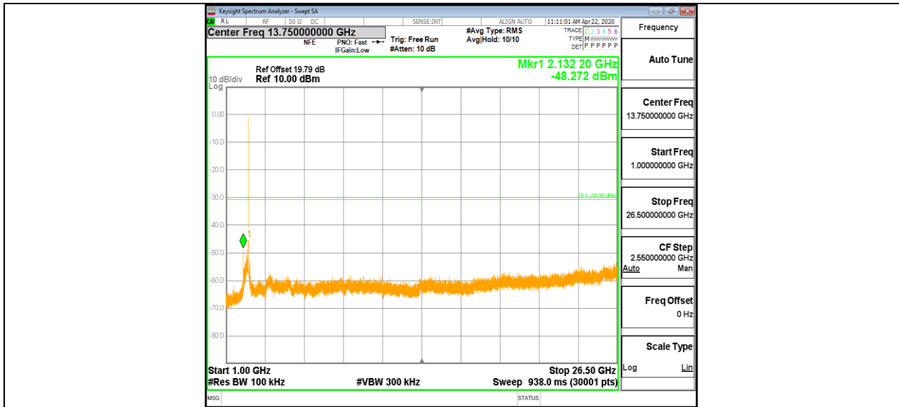
11N20MIMO_Ant2_2462_0~Reference
