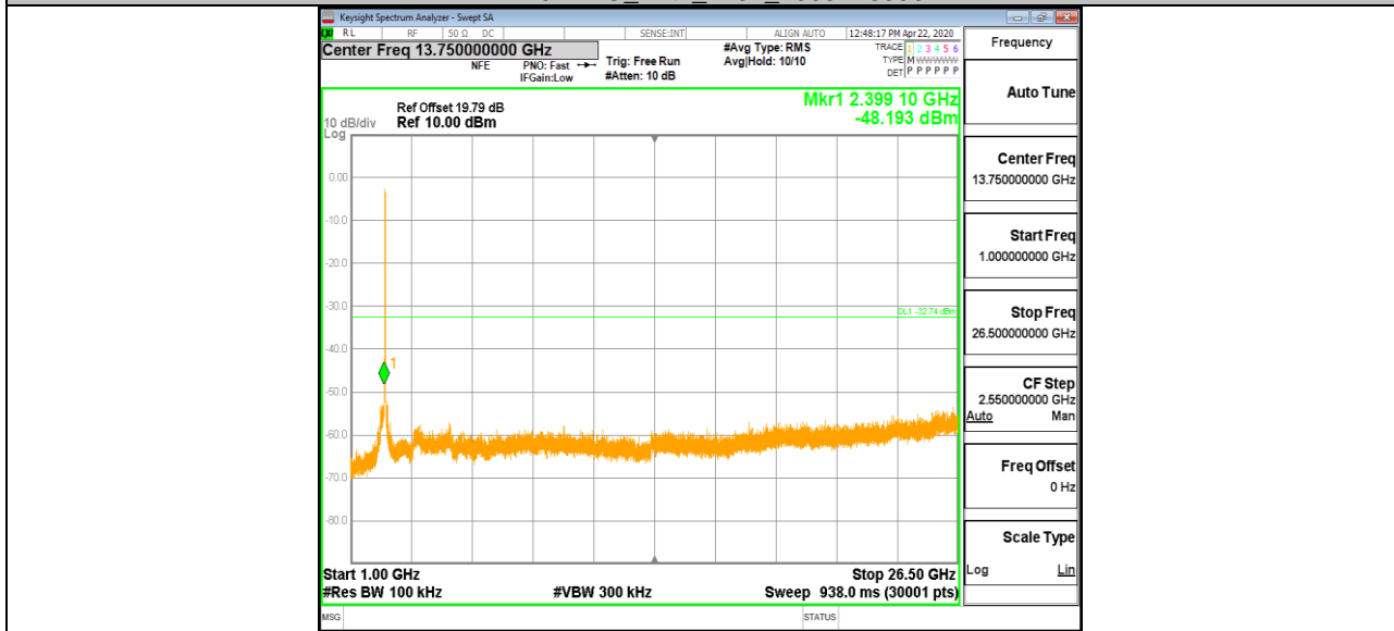
11N40MIMO_Ant1_2452_0~Reference
