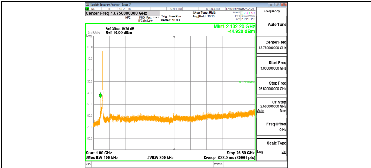
11N40MIMO_Ant2_2452_0~Reference
