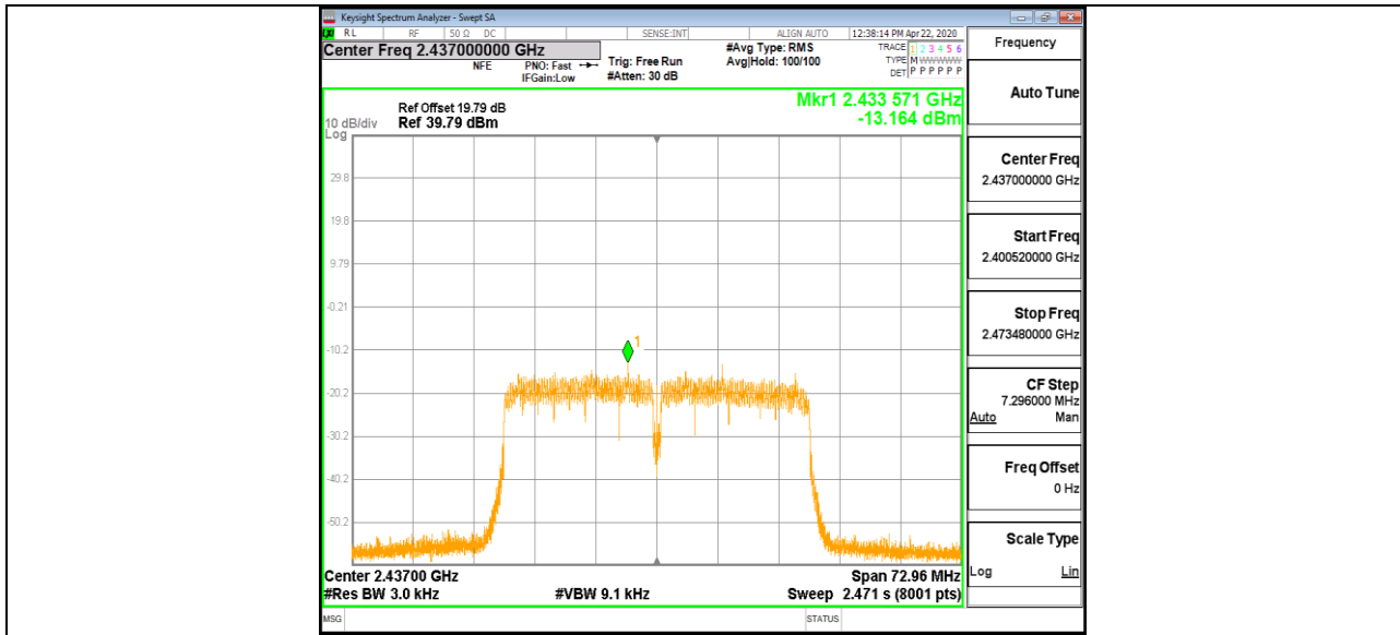
11N40MIMO_Ant2_2437
