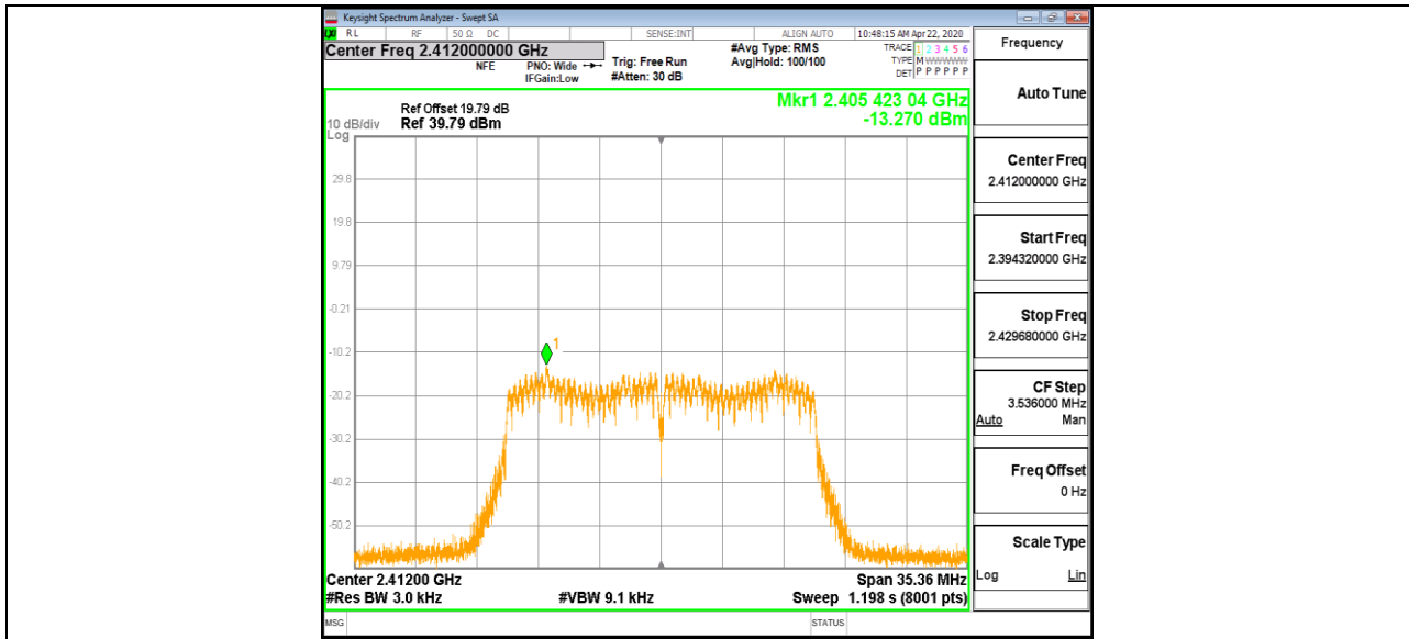
11N20MIMO_Ant2_2412
