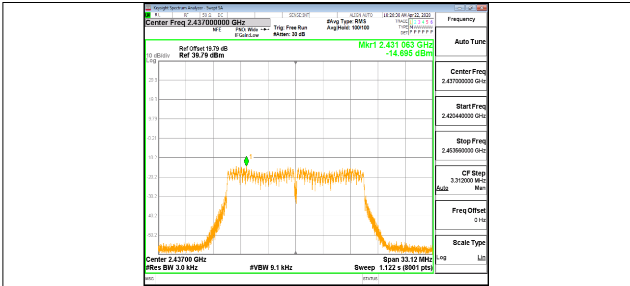
11G-MIMO_Ant2_2437
