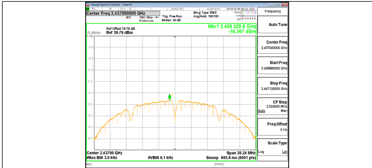
11B-MIMO_Ant2_2437
