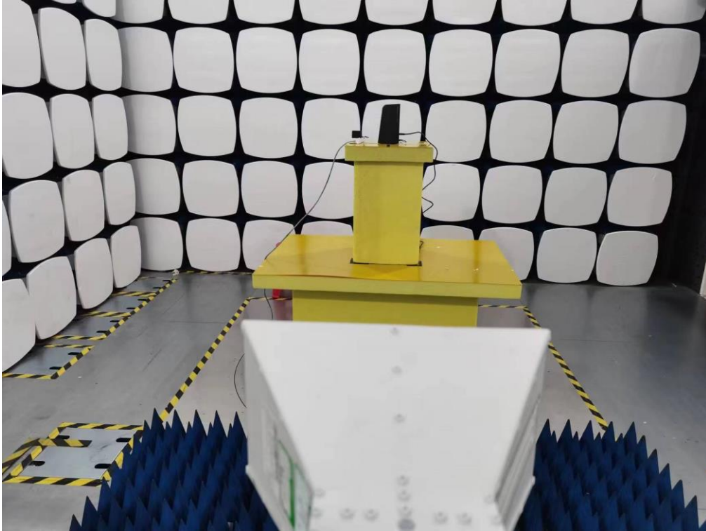
RSE (1-18) GHz
