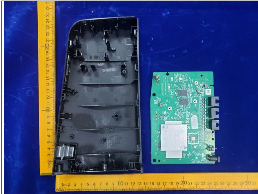
SR1021F EUT-2
