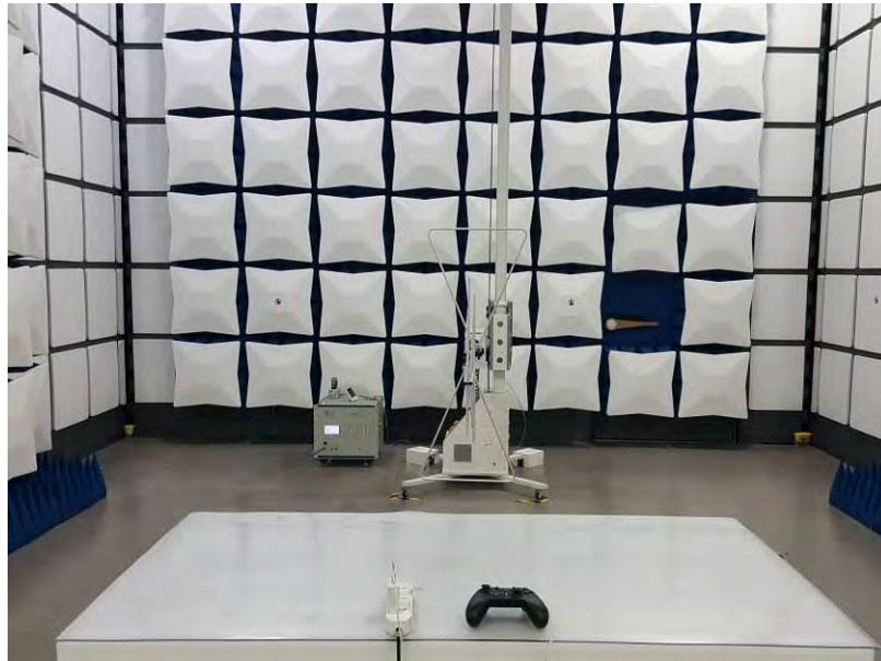
30MHz-1000MHz
