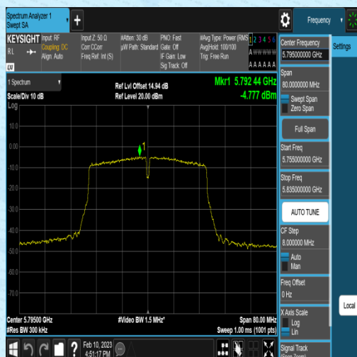
11N40MIMO-Ant1-5795--7.26-0.26-2.22-0.00
