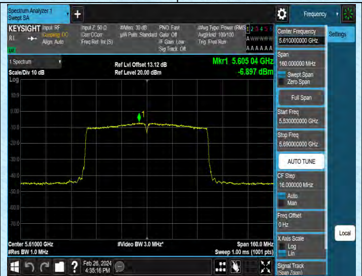
11AC80SISO-Ant2-5610-PASS
