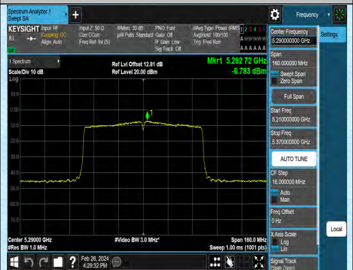
11AC80SISO-Ant2-5290-PASS
