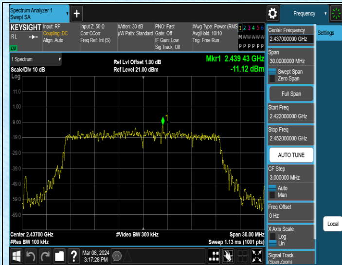
11AX20MIMO-Ant1-2437-0-Reference-PASS
