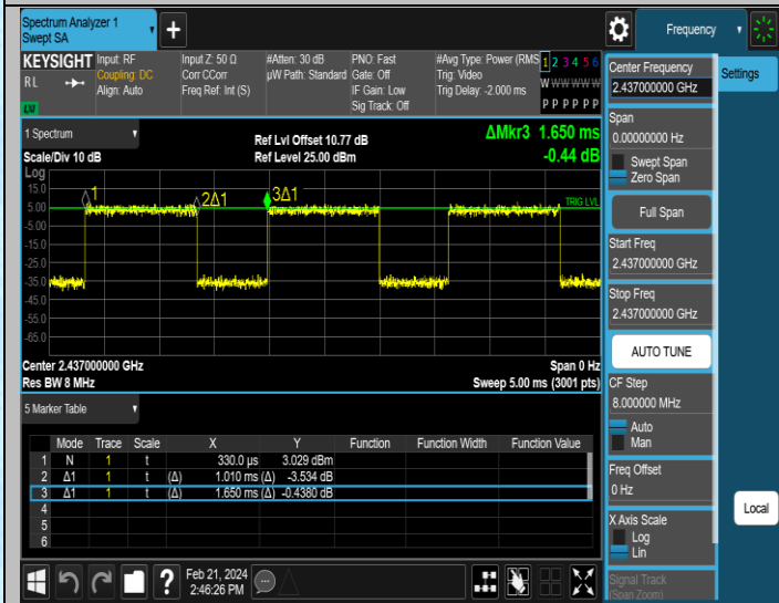
NTNV-11AX20MIMO-Ant1-2437
