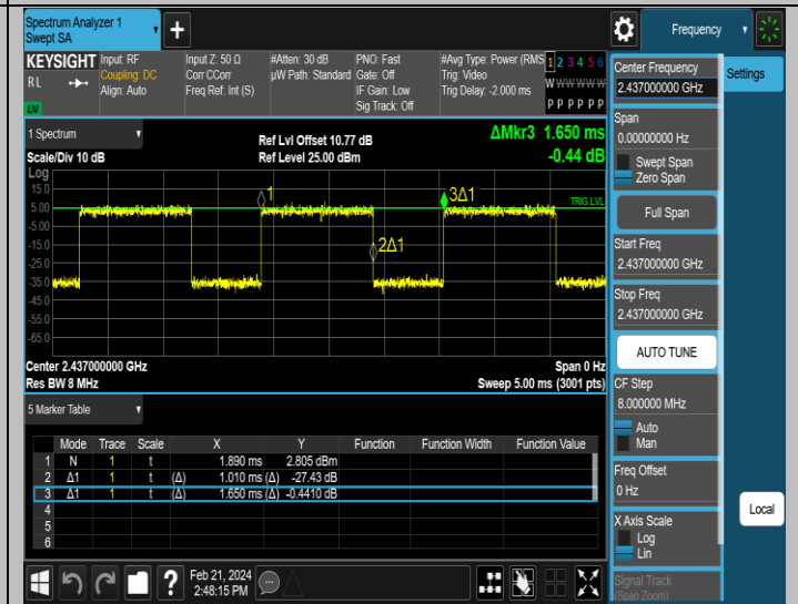
NTNV-11AX20MIMO-Ant2-2437
