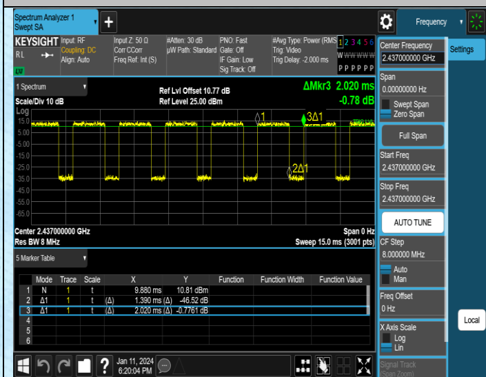
NTNV-11G-Ant1-2437
