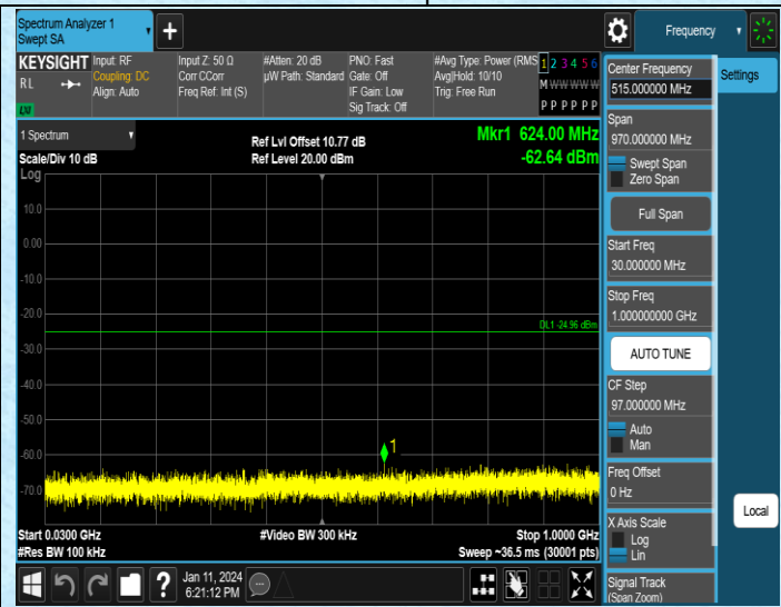
11G-Ant1-2437-30~1000-PASS
