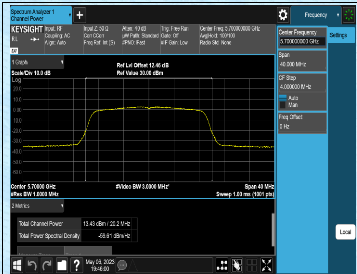
11N20MIMO-Ant1-5700
