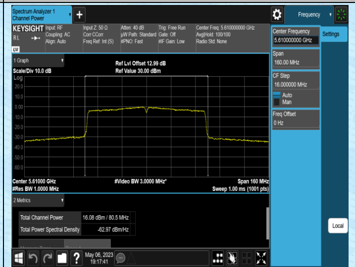
11AC80SISO-Ant2-5610
