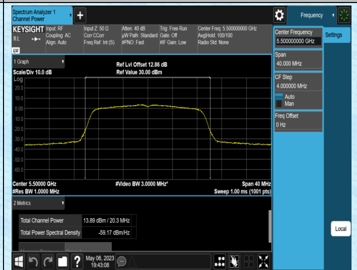
11N20MIMO-Ant2-5500
