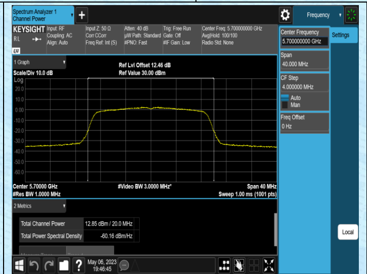
11N20MIMO-Ant2-5700
