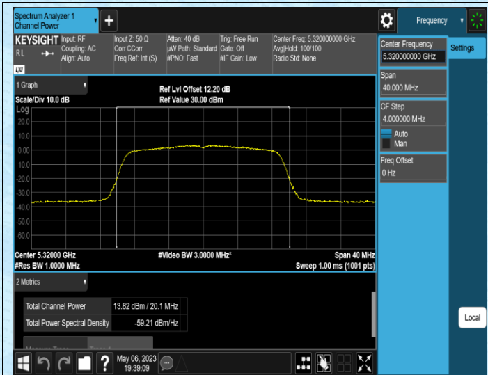
11N20MIMO-Ant1-5320
