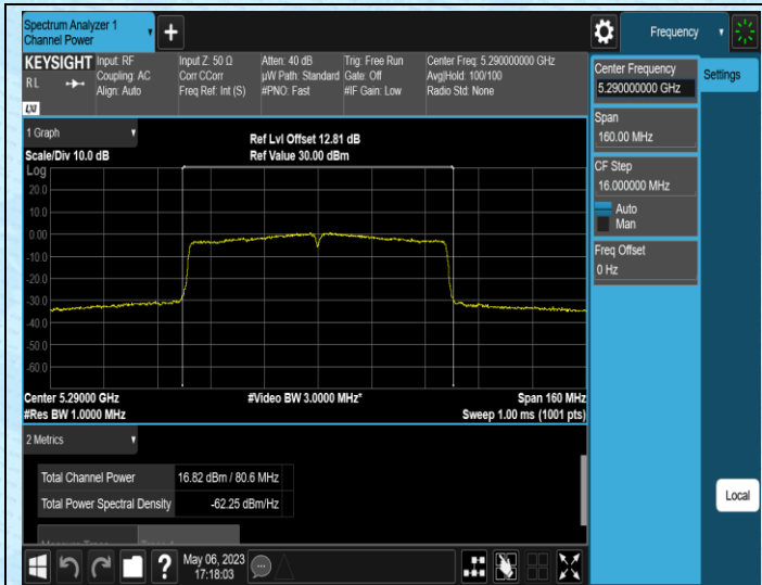
11AC80SISO-Ant1-5290
