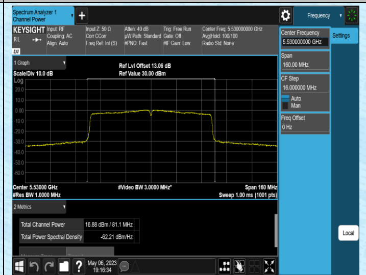
11AC80SISO-Ant2-5530
