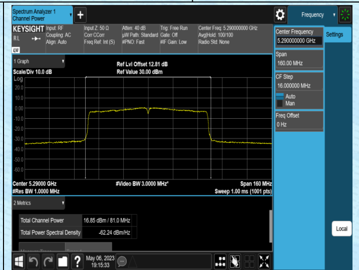
11AC80SISO-Ant2-5290
