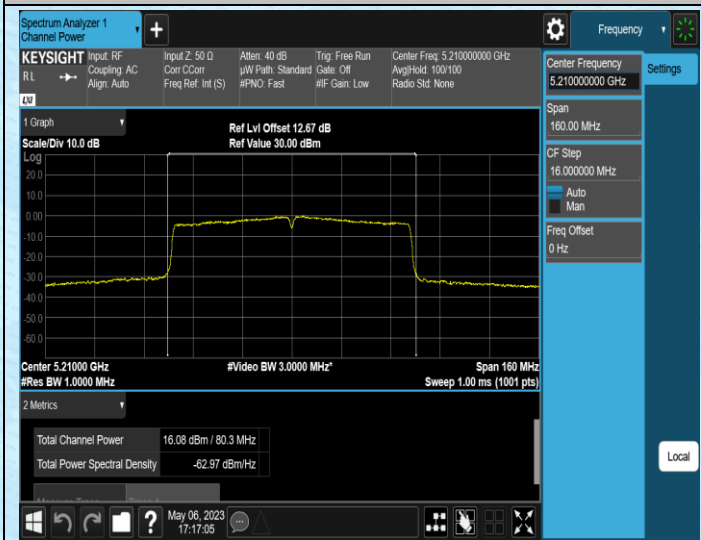
11AC80SISO-Ant1-5210
