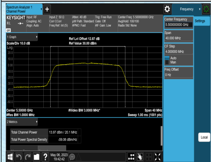
11N20MIMO-Ant1-5500
