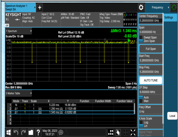
NTNV-11N20MIMO-Ant1-5280
