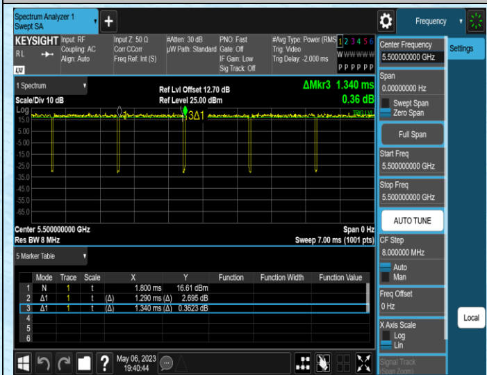
NTNV-11N20MIMO-Ant1-5500
