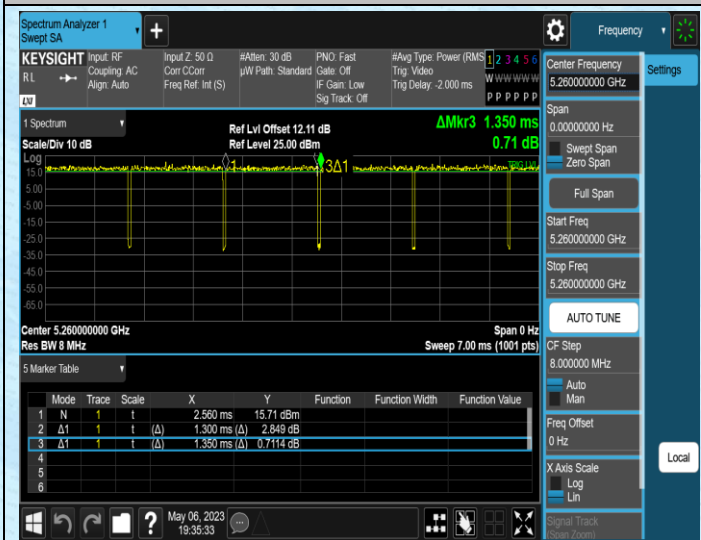
NTNV-11N20MIMO-Ant1-5260
