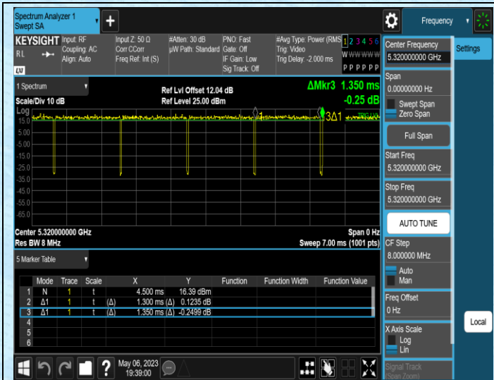
NTNV-11N20MIMO-Ant1-5320
