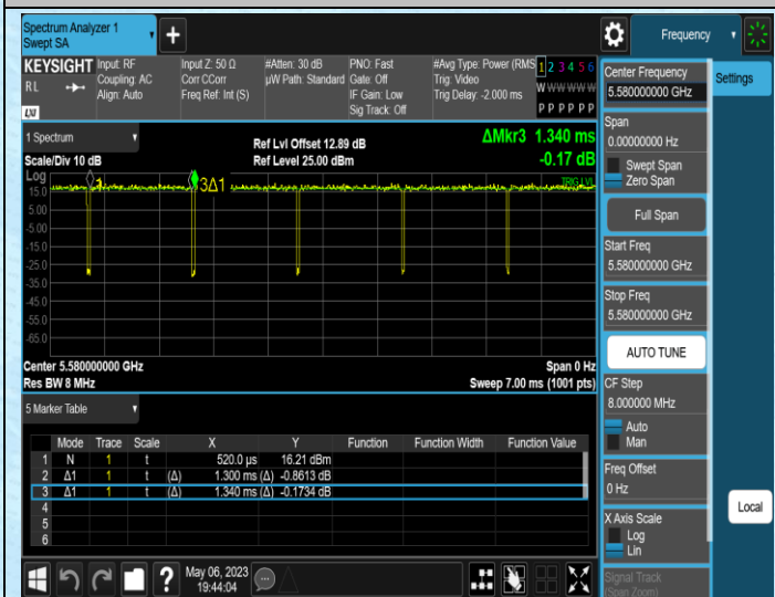
NTNV-11N20MIMO-Ant1-5580
