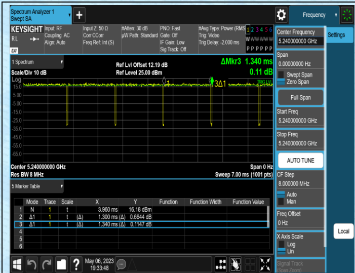
NTNV-11N20MIMO-Ant1-5240
