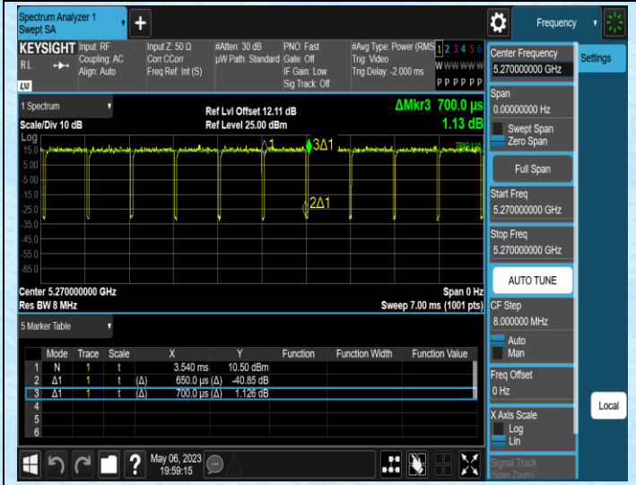
NTNV-11N40MIMO-Ant1-5270
