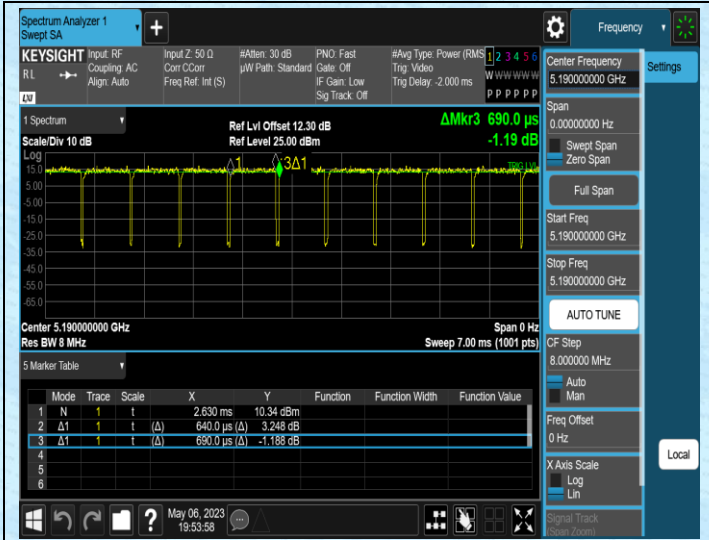
NTNV-11N40MIMO-Ant1-5190
