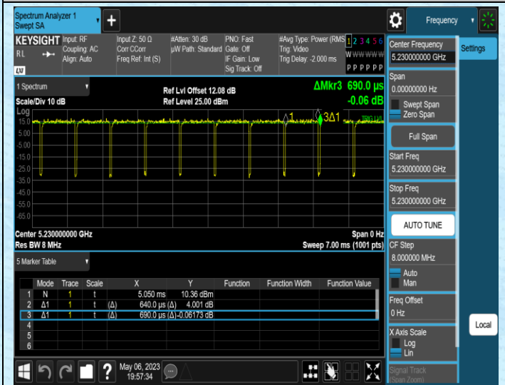
NTNV-11N40MIMO-Ant1-5230
