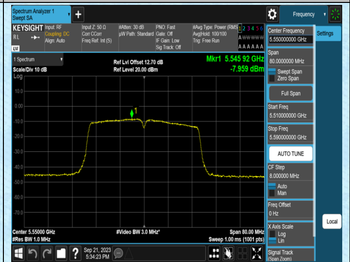
11AC40MIMO-Ant1-5550
