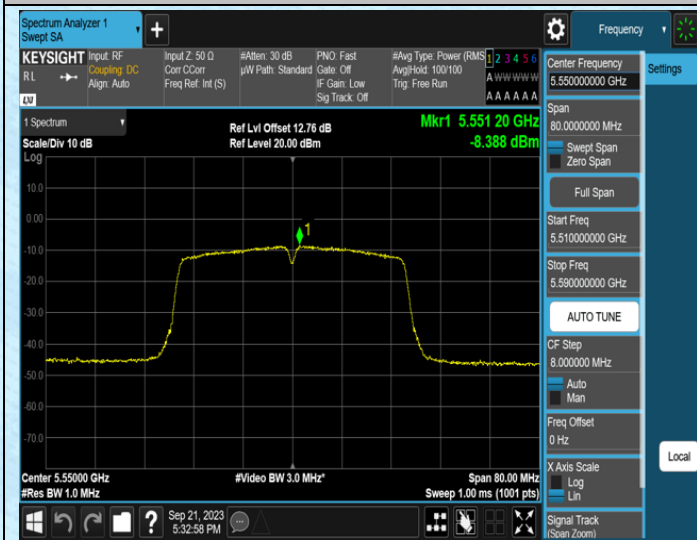
11AC40MIMO-Ant0-5550
