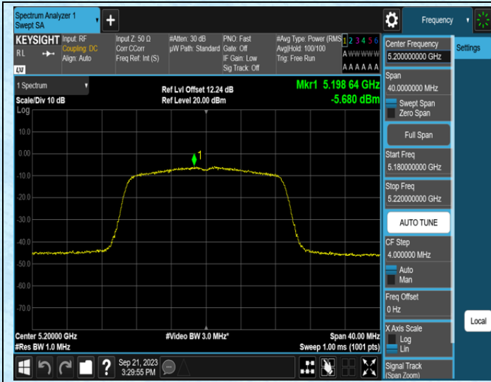
11N20MIMO-Ant0-5200
