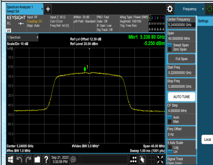
11N20MIMO-Ant0-5240
