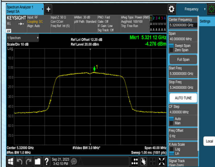
11N20MIMO-Ant0-5320
