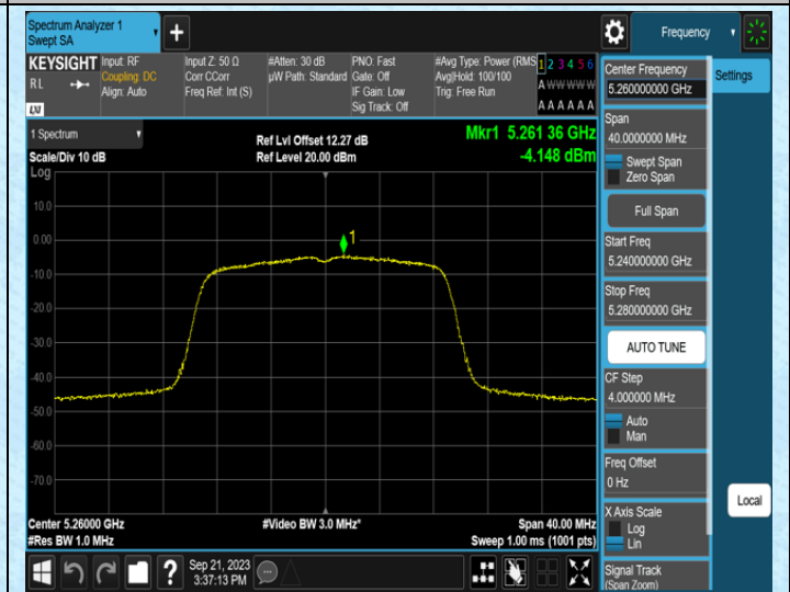
11N20MIMO-Ant1-5260
