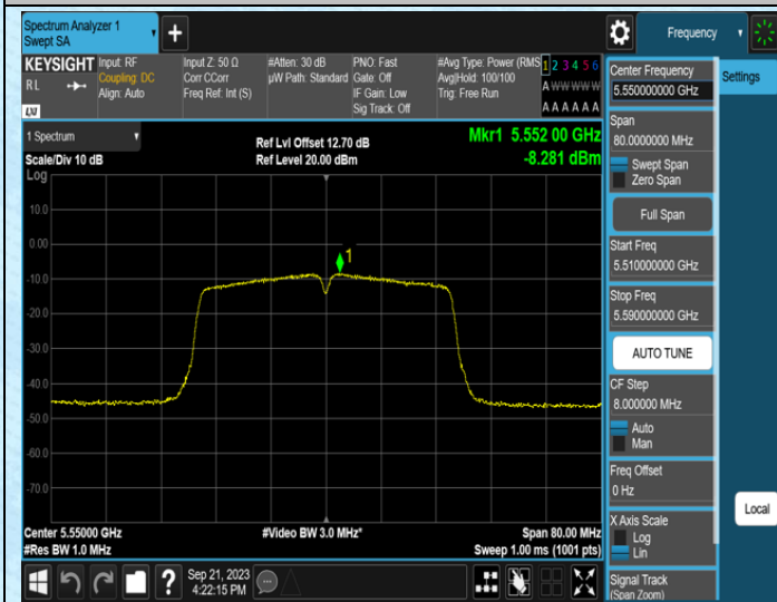
11N40MIMO-Ant0-5550
