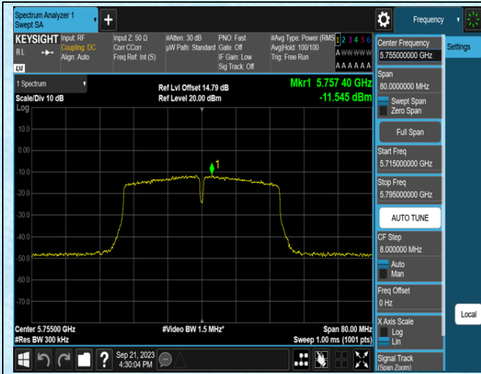
11N40MIMO-Ant0-5755
