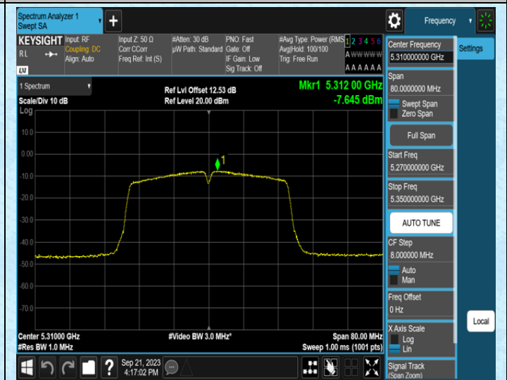
11N40MIMO-Ant1-5310
