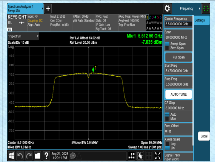
11N40MIMO-Ant1-5510
