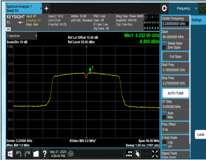
11N40MIMO-Ant0-5230
