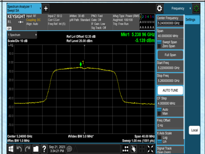
11N20MIMO-Ant1-5240
