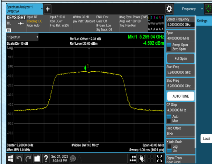
11N20MIMO-Ant0-5260
