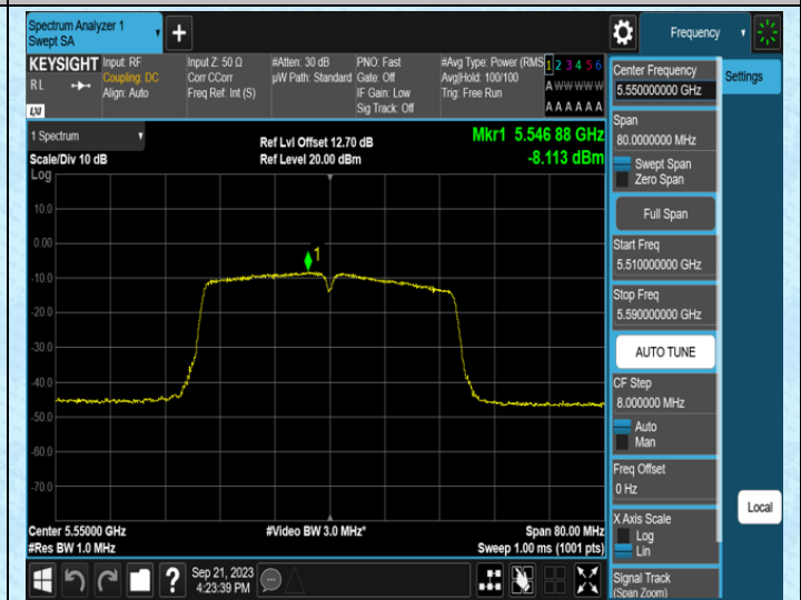
11N40MIMO-Ant1-5550
