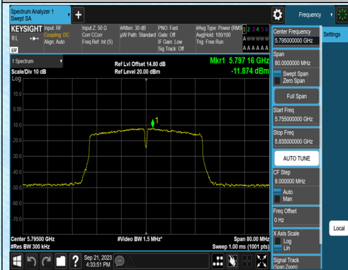
11N40MIMO-Ant0-5795
