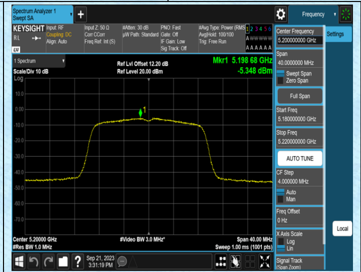
11N20MIMO-Ant1-5200
