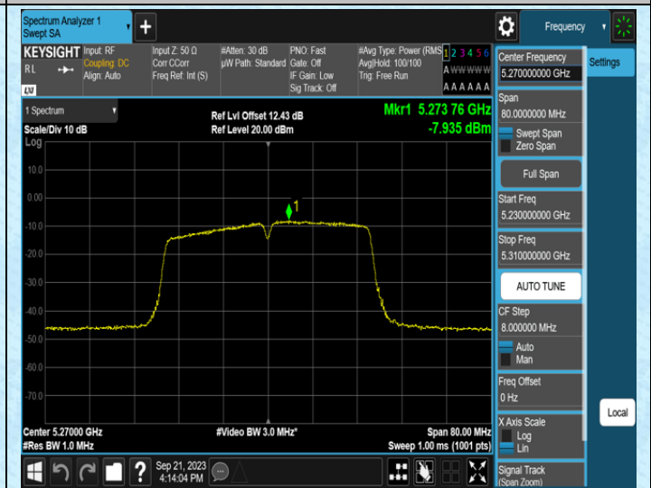
11N40MIMO-Ant1-5270
