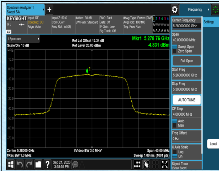
11N20MIMO-Ant0-5280
