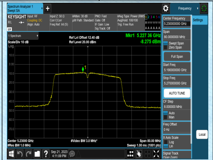
11N40MIMO-Ant1-5230
