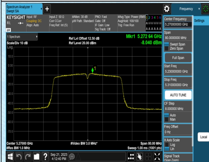
11N40MIMO-Ant0-5270
