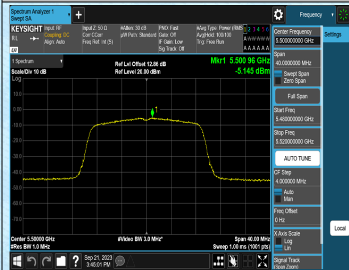
11N20MIMO-Ant0-5500
