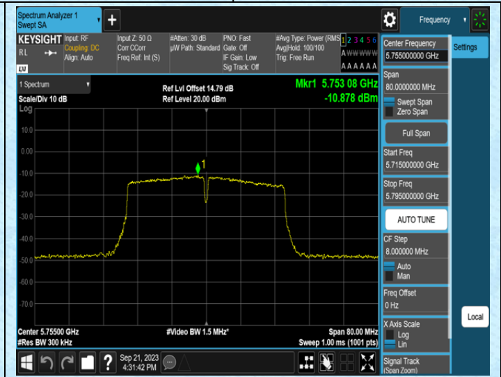
11N40MIMO-Ant1-5755
