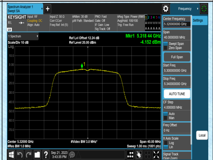
11N20MIMO-Ant1-5320
