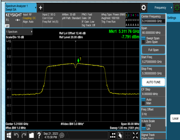
11N40MIMO-Ant0-5310
