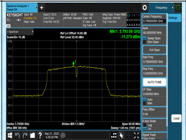
11N40MIMO-Ant1-5795
