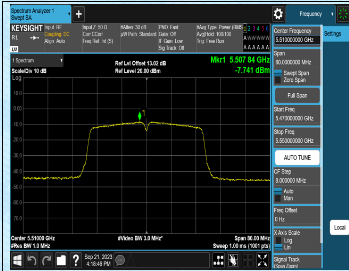
11N40MIMO-Ant0-5510
