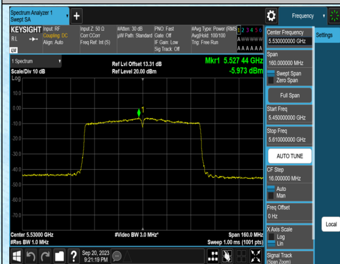
11AC80SISO-Ant0-5530
