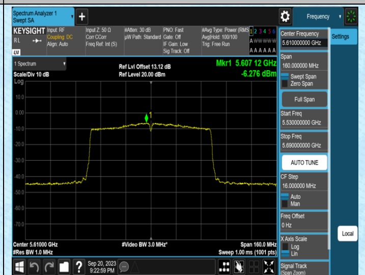
11AC80SISO-Ant0-5610
