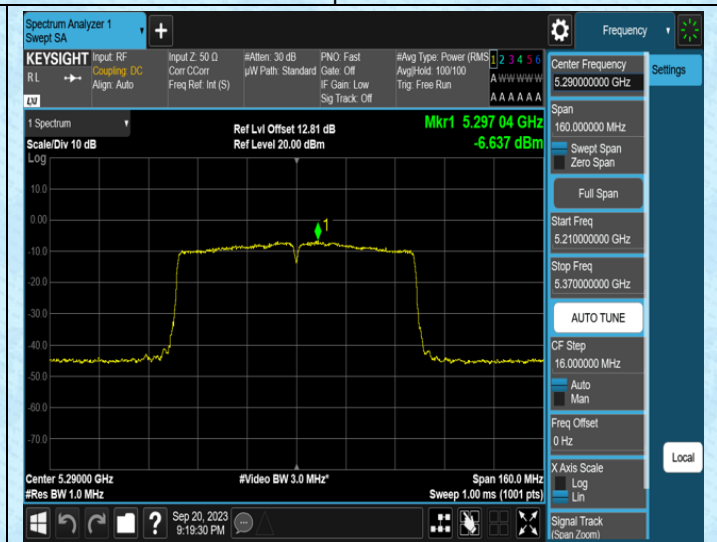
11AC80SISO-Ant0-5290
