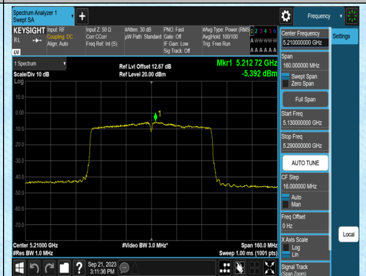
11AC80SISO-Ant1-5210
