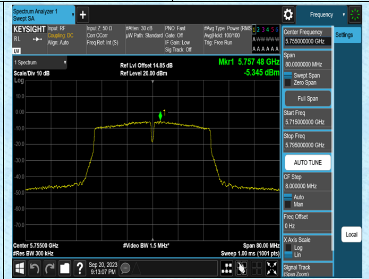
11AC40SISO-Ant0-5755
