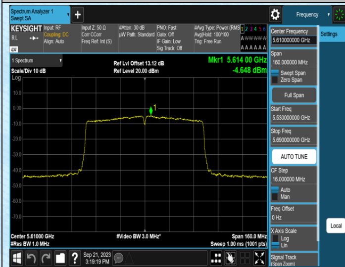
111AC80SISO-Ant1-5610
