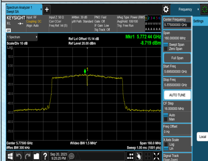
11AC80SISO-Ant0-5775
