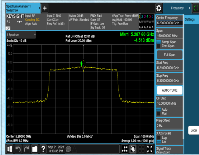
111AC80SISO-Ant1-5290
