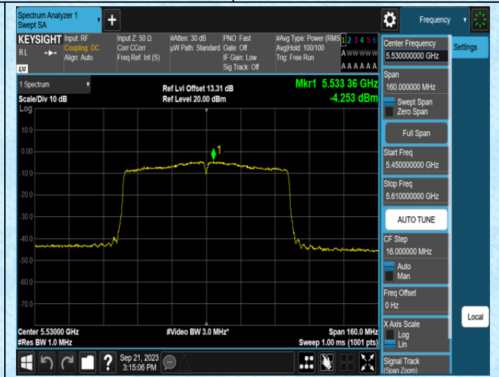
111AC80SISO-Ant1-5530
