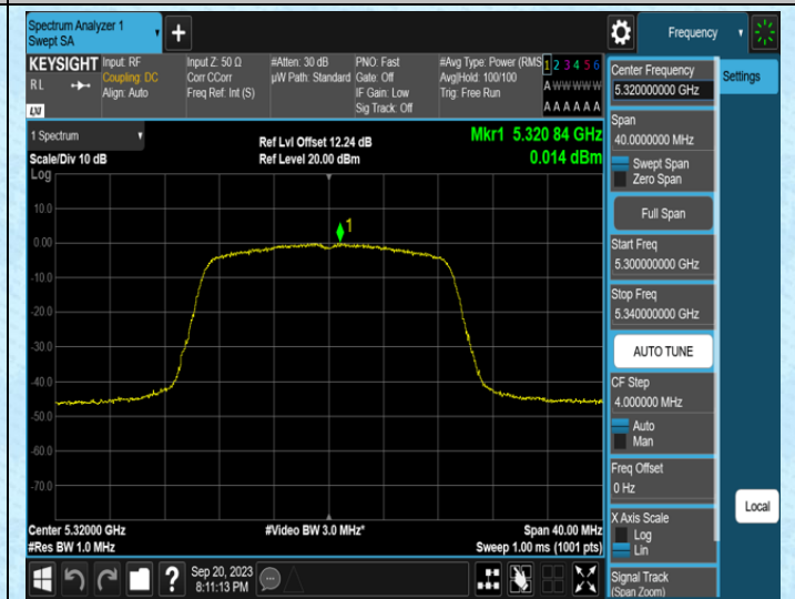
11N20SISO-Ant0-5320
