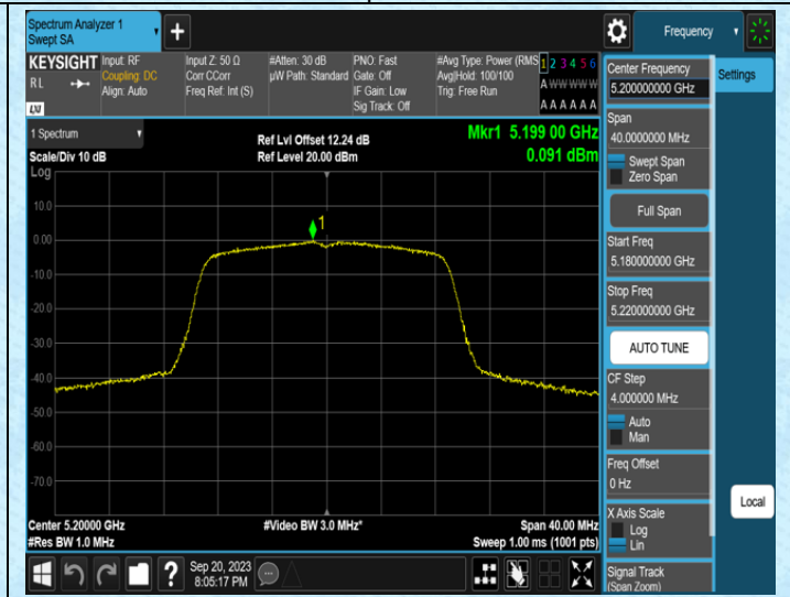
11N20SISO-Ant0-5200
