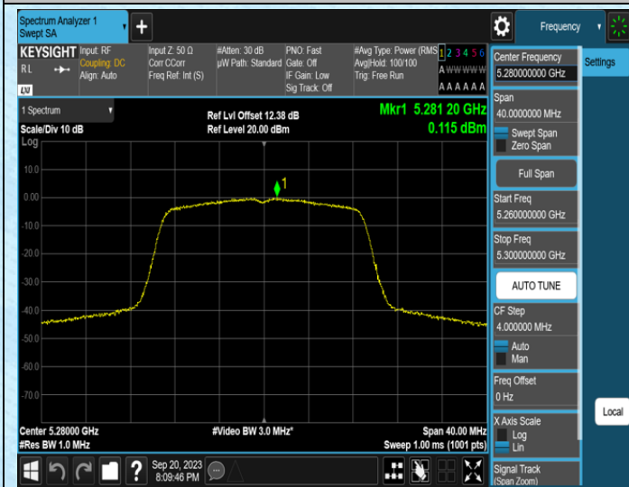
11N20SISO-Ant0-5280
