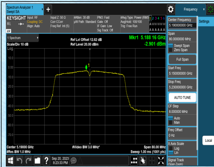
11N40SISO-Ant0-5190
