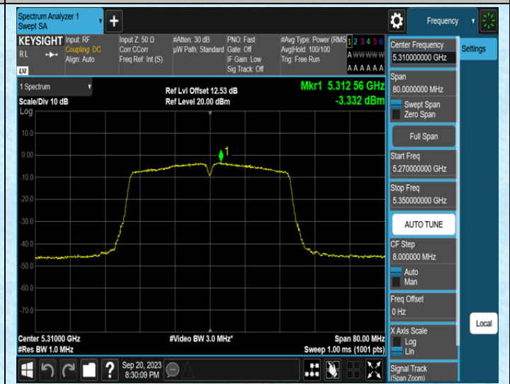
11N40SISO-Ant0-5310
