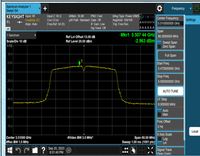
11N40SISO-Ant0-5510
