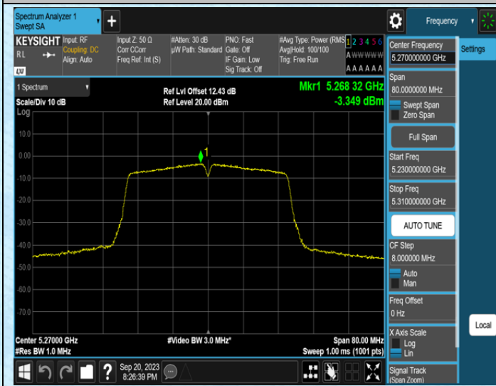
11N40SISO-Ant0-5270
