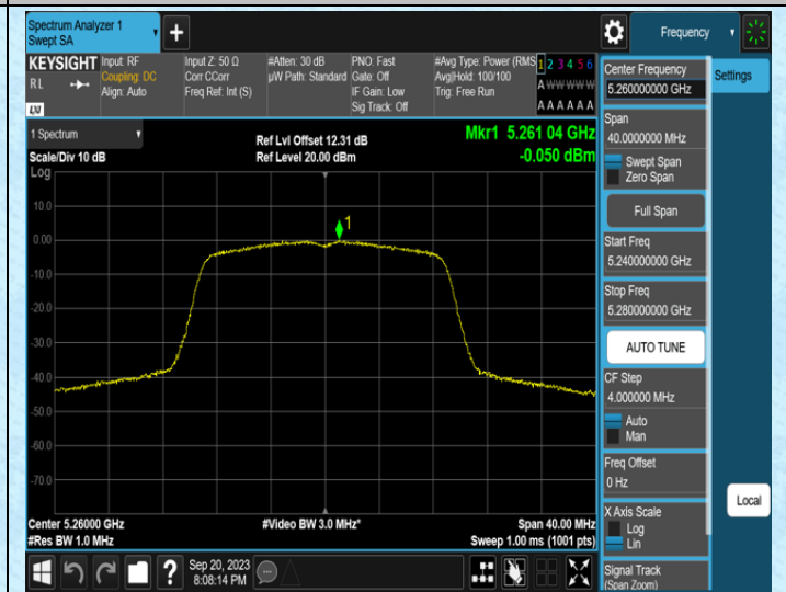
11N20SISO-Ant0-5260
