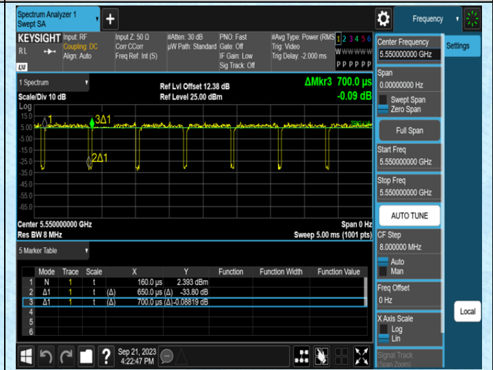
NTNV-11N40MIMO-Ant1-5550
