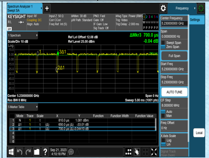
NTNV-11N40MIMO-Ant1-5230
