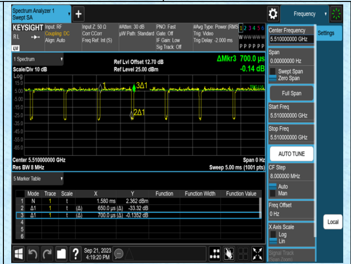
NTNV-11N40MIMO-Ant1-5510
