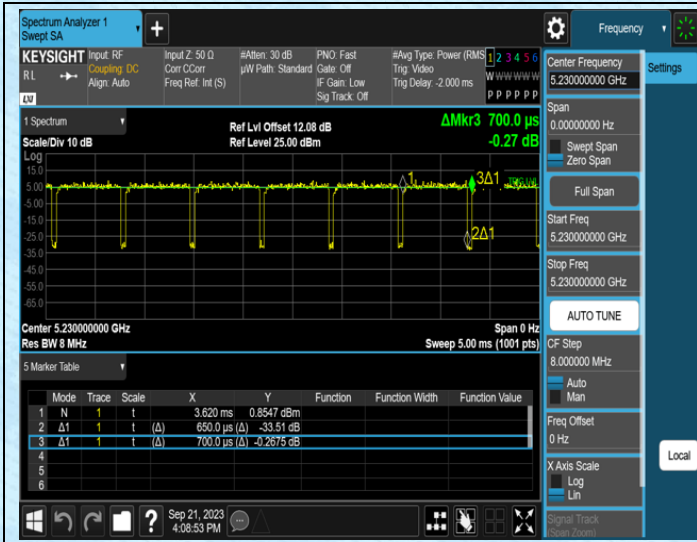
NTNV-11N40MIMO-Ant0-5230
