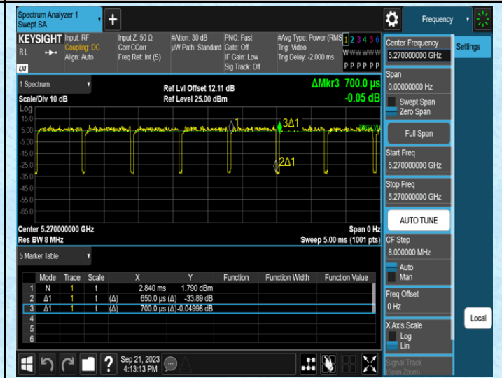
NTNV-11N40MIMO-Ant1-5270
