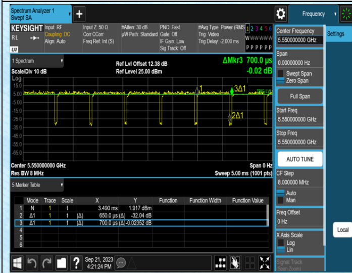
NTNV-11N40MIMO-Ant0-5550
