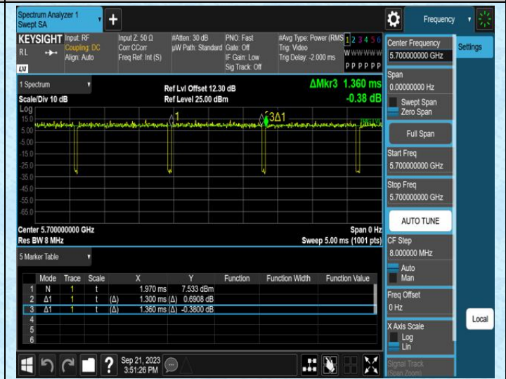
NTNV-11N20MIMO-Ant1-5700
