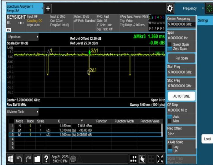
NTNV-11AC20MIMO-Ant0-5700
