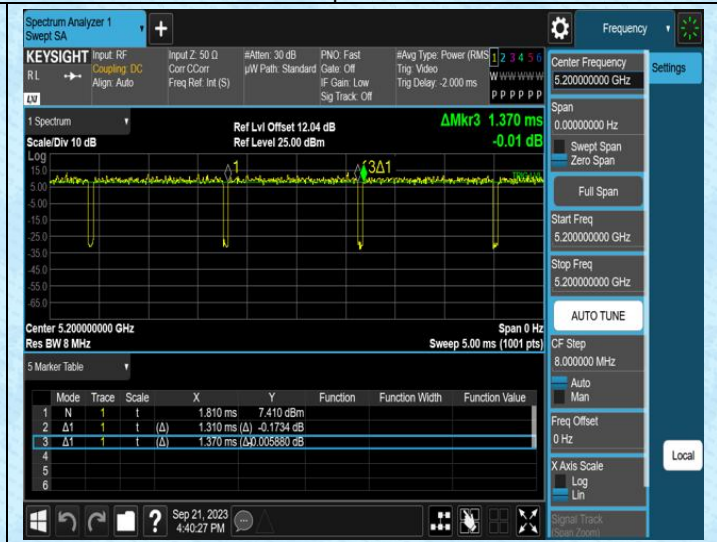
NTNV-11AC20MIMO-Ant1-5200
