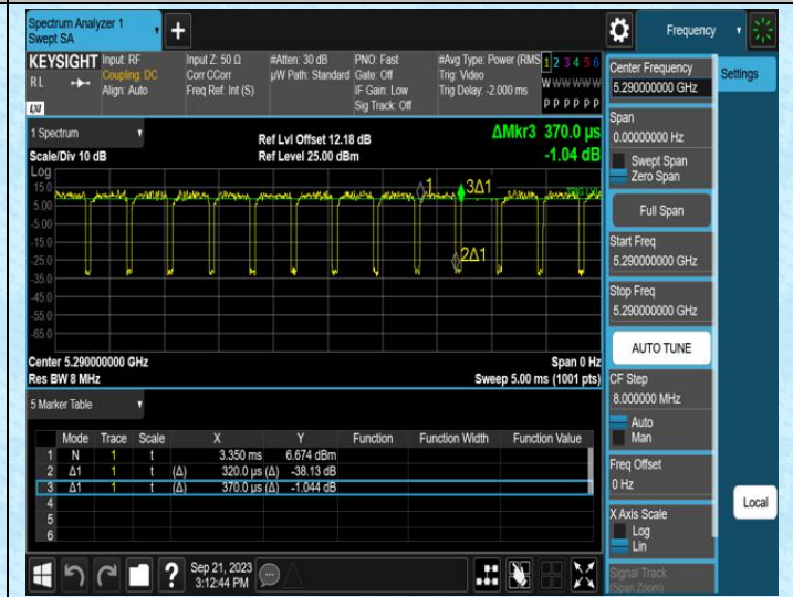
NTNV-11AC80SISO-Ant1-5290
