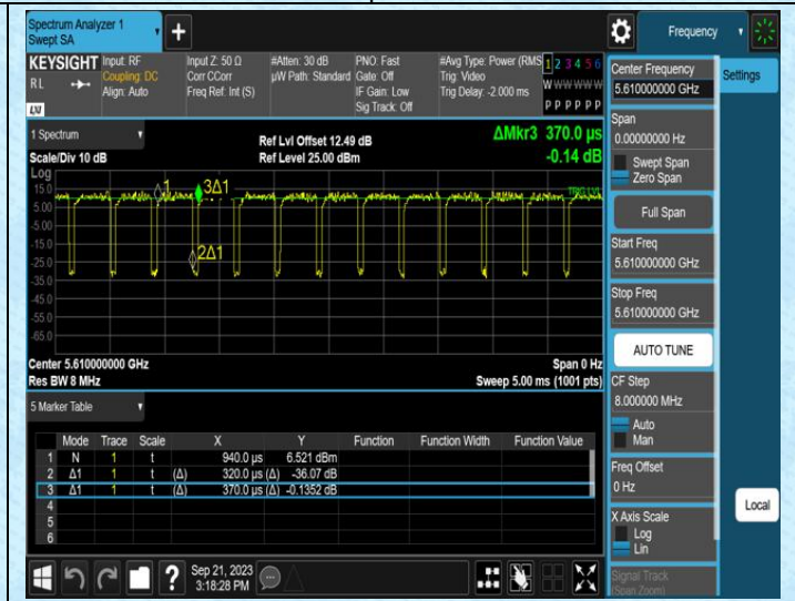
NTNV-11AC80SISO-Ant1-5610
