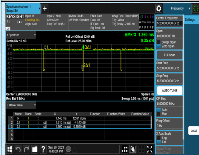
NTNV-11AC20SISO-Ant0-5200
