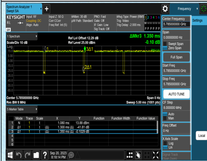
NTVN-11N20SISO-Ant0-5785
