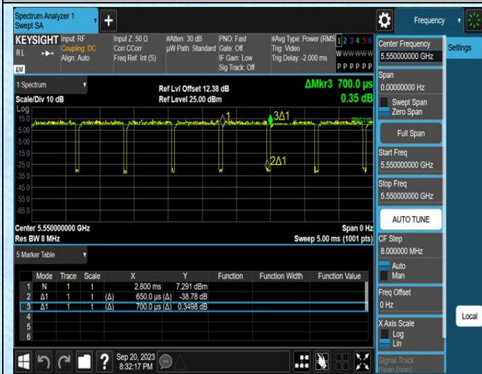
NTVN-11N40SISO-Ant0-5550
