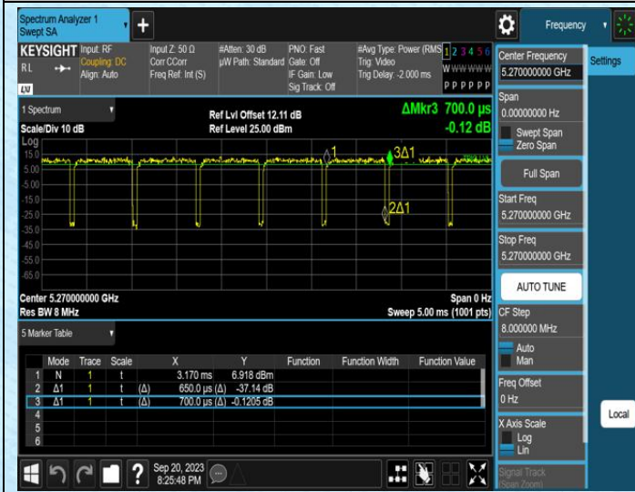
NTVN-11N40SISO-Ant0-5270
