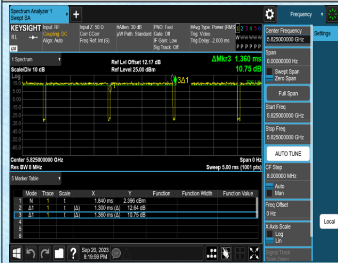
NTVN-11N20SISO-Ant0-5825
