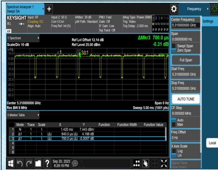
NTVN-11N40SISO-Ant0-5310
