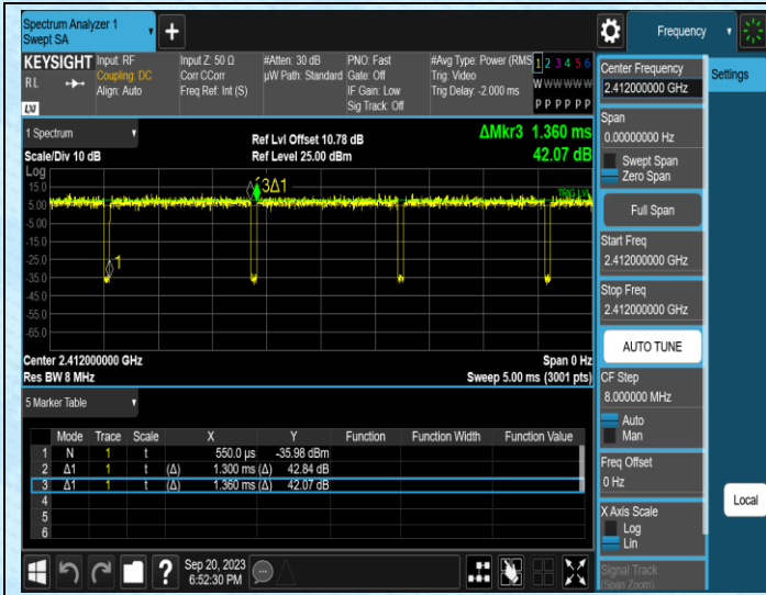
NTNV-11N20MIMO-Ant0-2412
