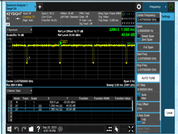
NTNV-11N20MIMO-Ant1-2437
