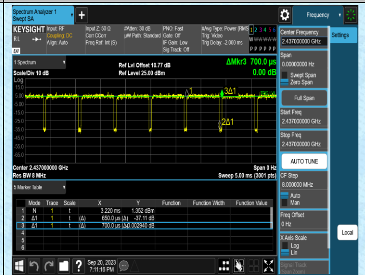
NTNV-11N40MIMO-Ant1-2437
