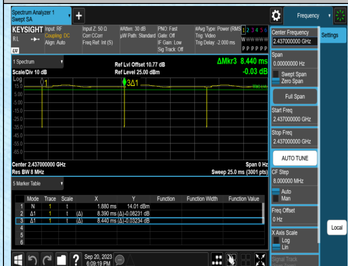
NTNV-11B-Ant0-2437
