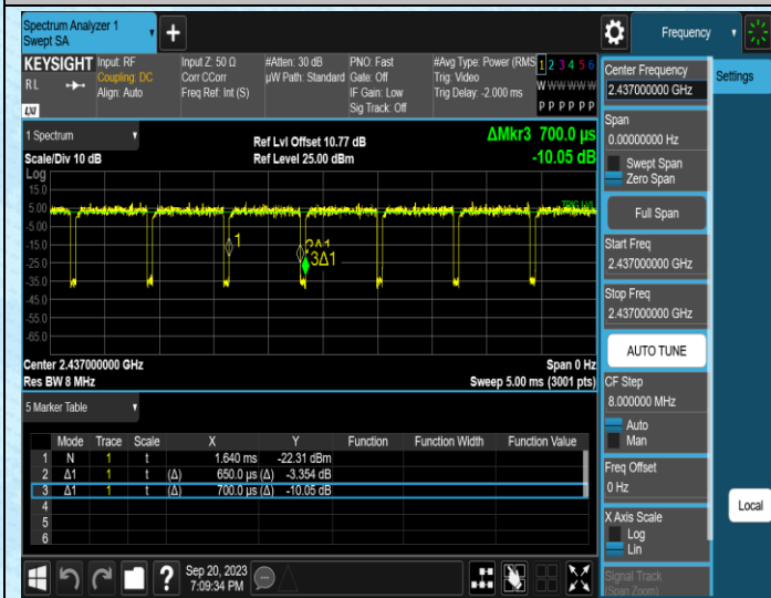
NTNV-11N40MIMO-Ant0-2437
