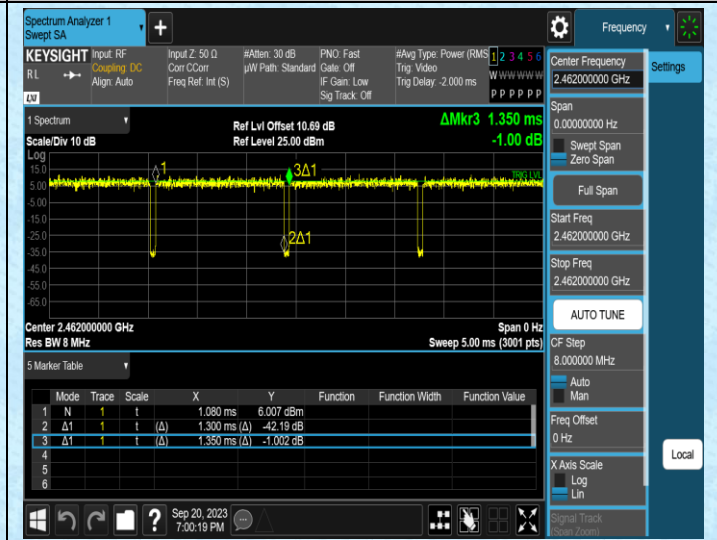
NTNV-11N20MIMO-Ant1-2462
