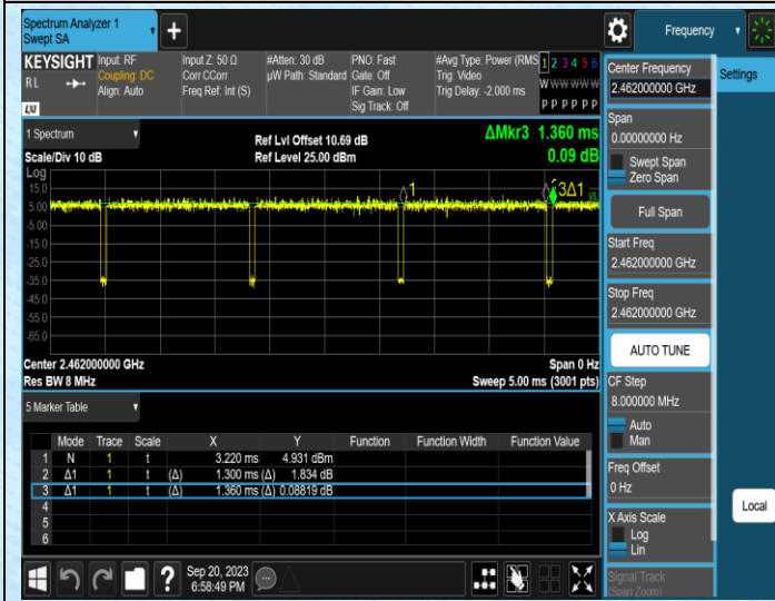
NTNV-11N20MIMO-Ant0-2462
