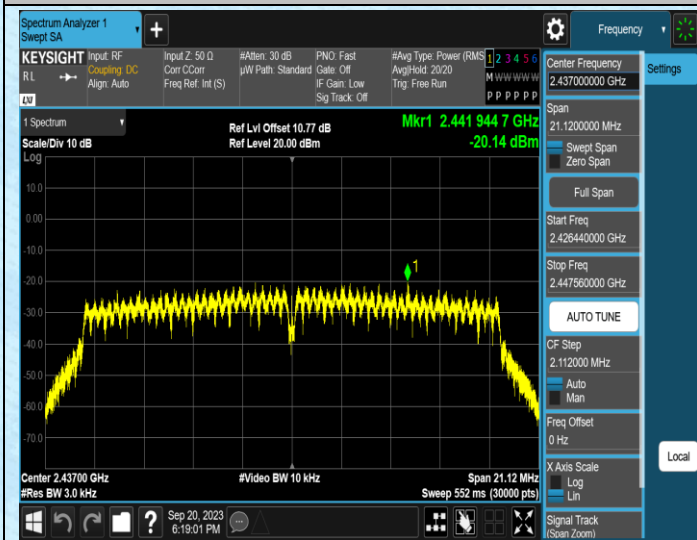
11N20SISO-Ant0-2437
