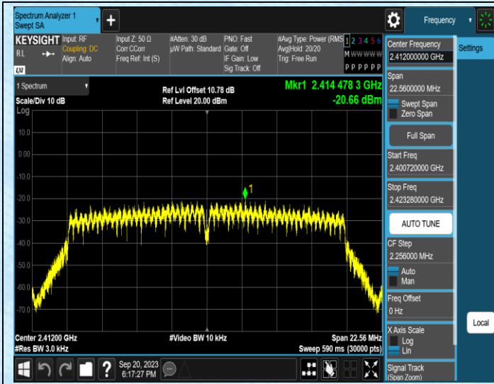
11N20SISO-Ant0-2412
