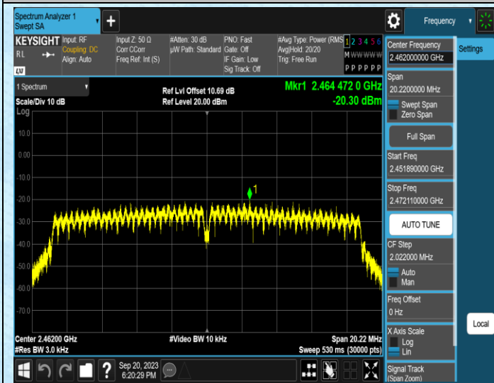
11N20SISO-Ant0-2462
