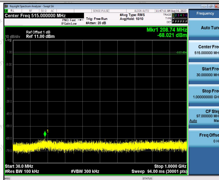
2.4G_Ant1_2442_30~1000
