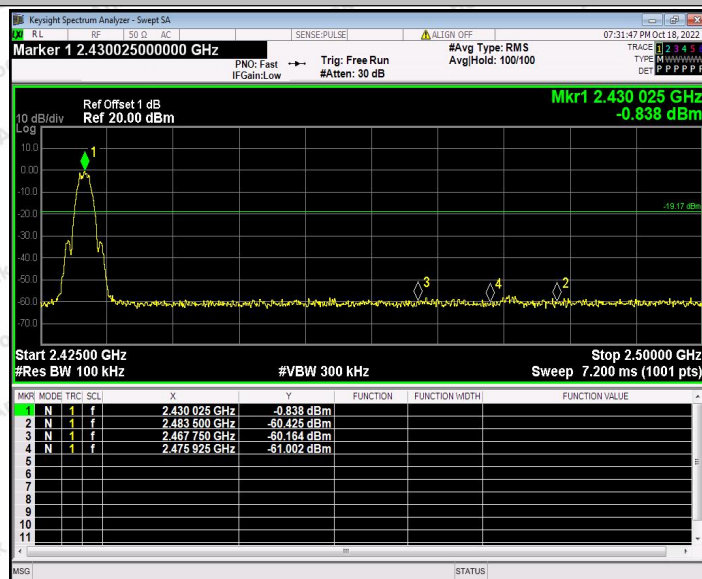
2.4g_Ant1_Low_2430
