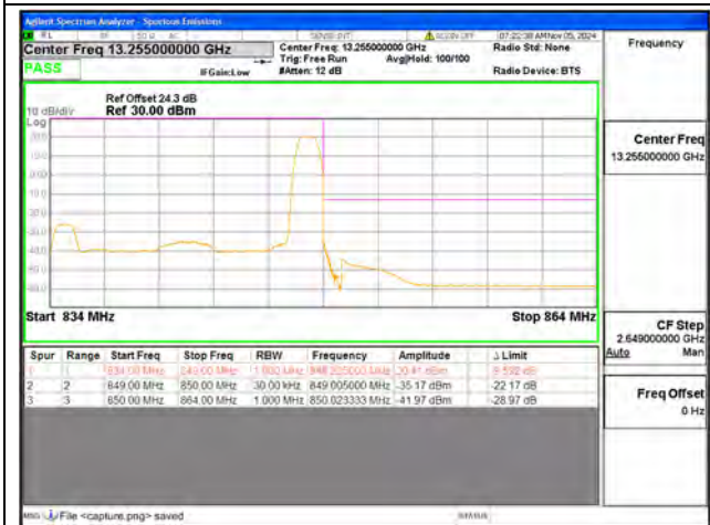
B26 / 15MHz / High CH / QPSK / 1 RB
