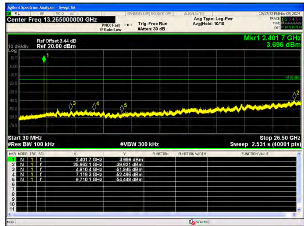
Tx. Spurious NVNT BLE 1M 2402MHz Ant1 Emission SISO
