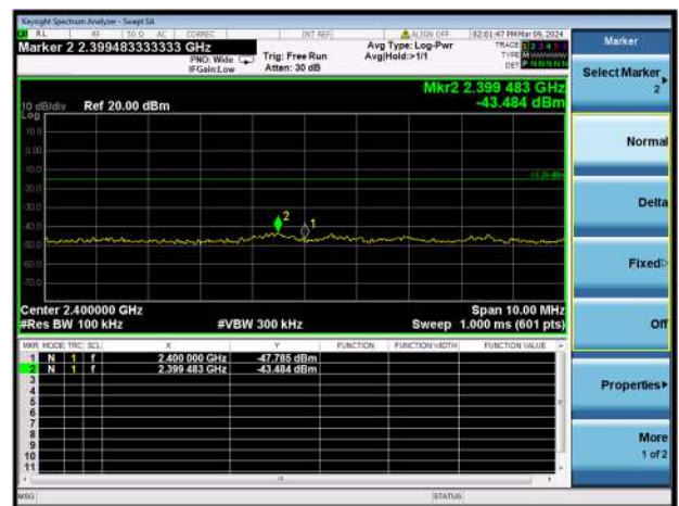
802.11b CH3, BAND EDGE
