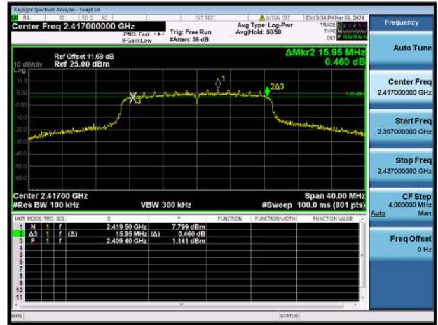
802.11n-20 MHz CH2
