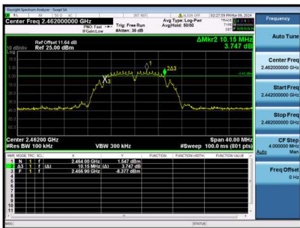
802.11b CH11
