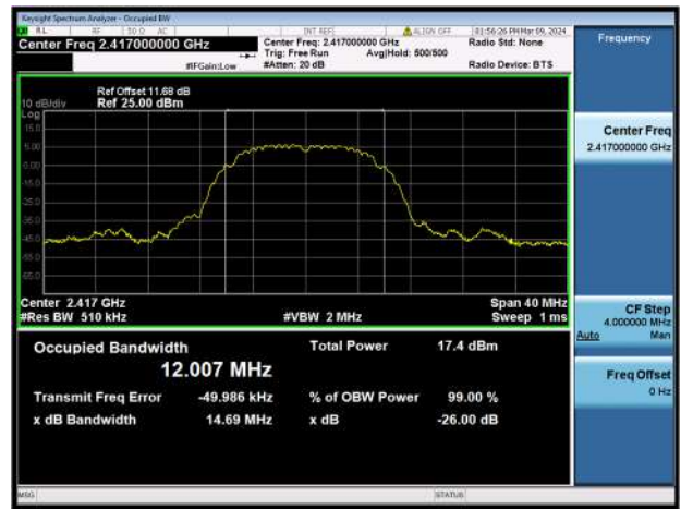
802.11b CH2
