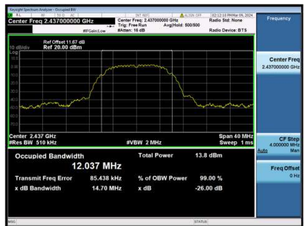
802.11b CH6
