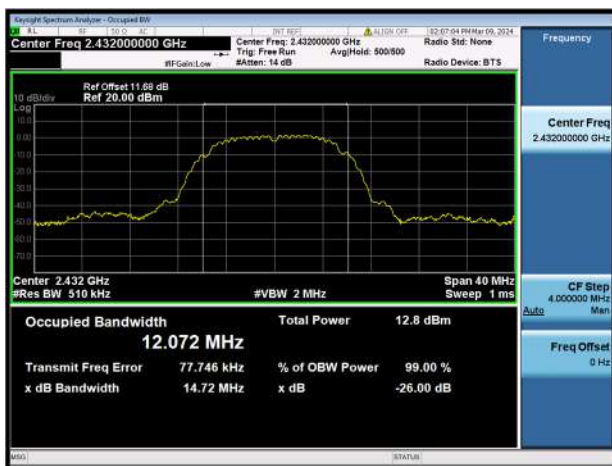
802.11b CH5
