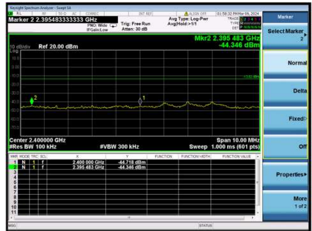
802.11b CH2, BAND EDGE
