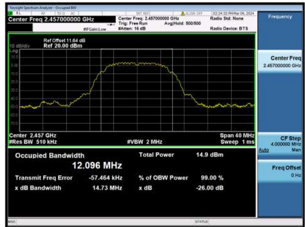
802.11b CH10
