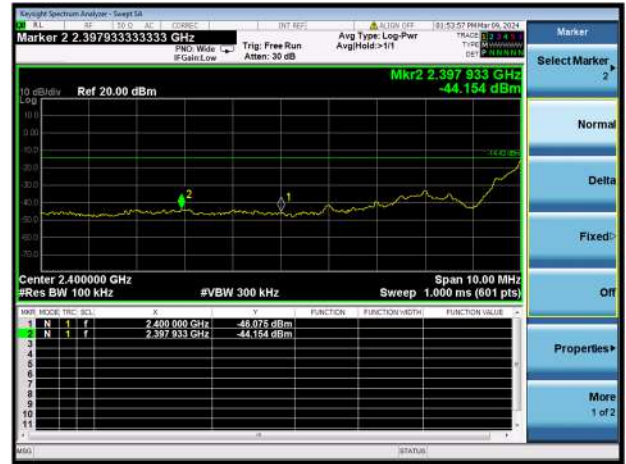
802.11b CH1, BAND EDGE
