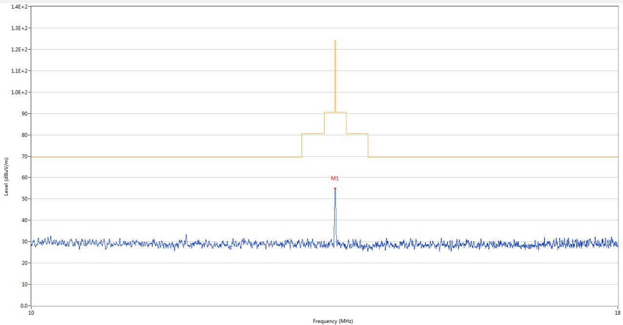
Test Antenna-LOOP, EUT Horizontal
