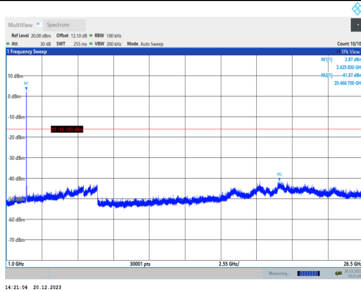
11AX40MIMO_Ant1_2437_242Tone_RU61_0~Reference
