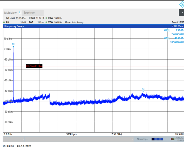
11AX20MIMO_Ant2_2412_106Tone_RU53_0~Reference
