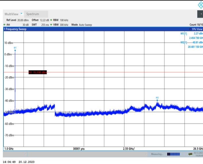
11AX40MIMO_Ant1_2422_26Tone_RU0_0~Reference
