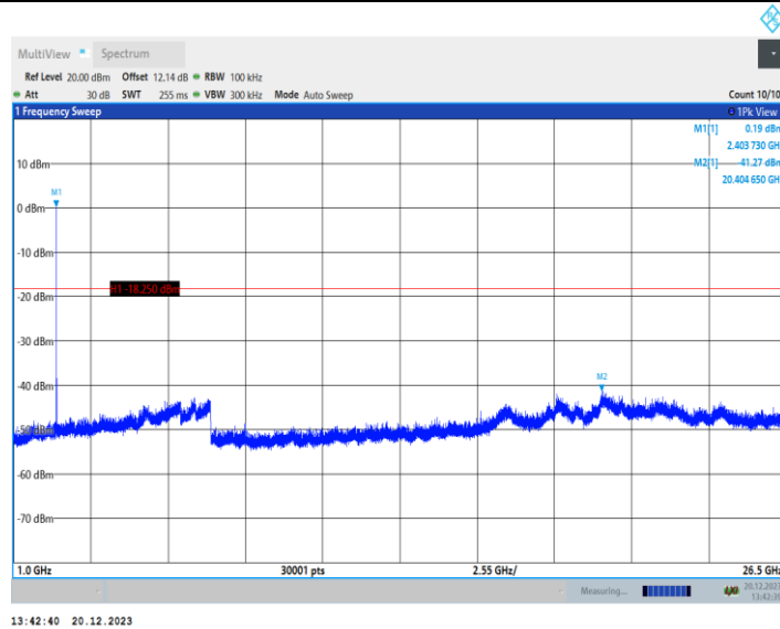
11AX20MIMO_Ant2_2412_52Tone_RU37_0-Reference
