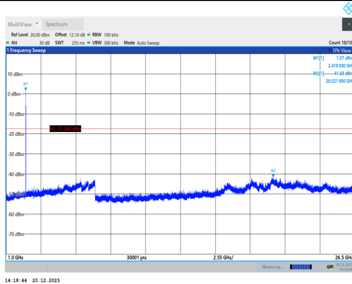
11AX40MIMO_Ant1_2437_52Tone_RU37_0-Reference
