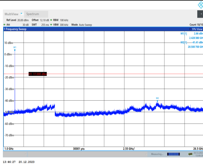
11AX20MIMO_Ant1_2437_52Tone_RU37_0-Reference
