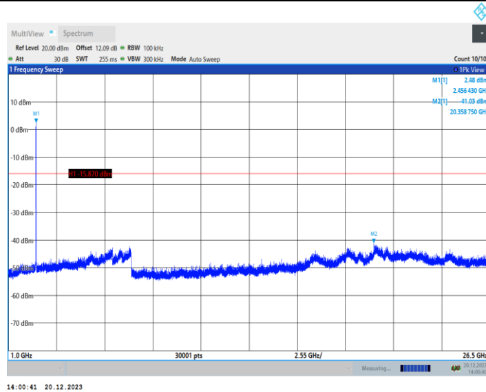
11AX20MIMO_Ant2_2462_26Tone_RU0_0~Reference
