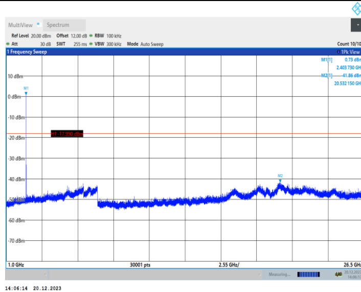
11AX40MIMO_Ant1_2422_52Tone_RU37_0-Reference
