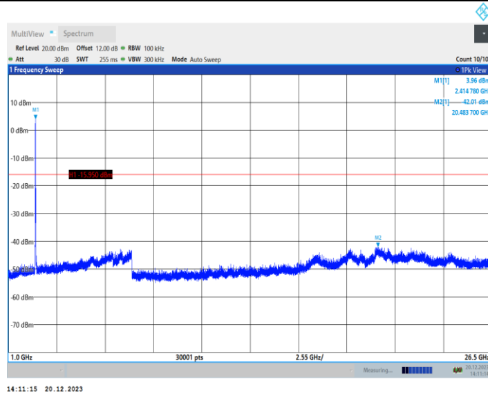
11AX40MIMO_Ant2_2422_26Tone_RU0_0~Reference
