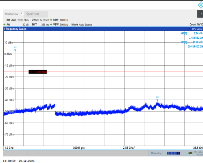
11AX20MIMO_Ant1_2462_106Tone_RU53_0~Reference
