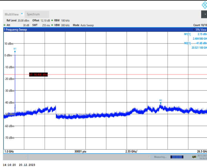
11AX40MIMO_Ant2_2422_242Tone_RU61_0~Reference
