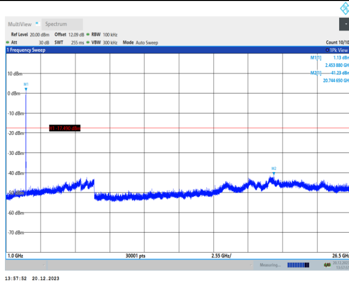
11AX20MIMO_Ant1_2462_52Tone_RU37_0-Reference
