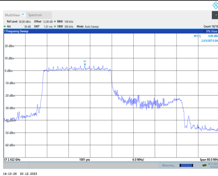
11AX40MIMO_Ant1_2422_242Tone_RU61_30~1000
