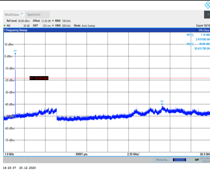
11AX40MIMO_Ant2_2437_52Tone_RU37_0-Reference
