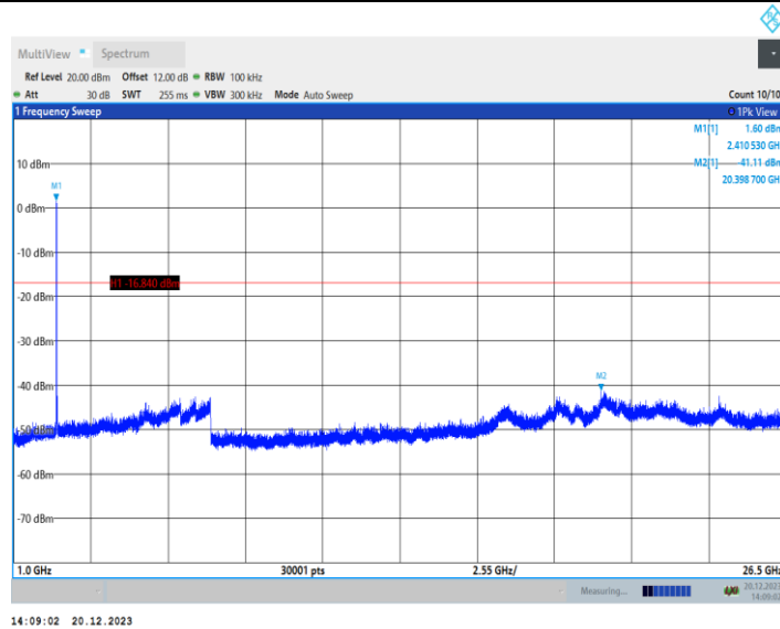
11AX40MIMO_Ant1_2422_242Tone_RU61_0~Reference
