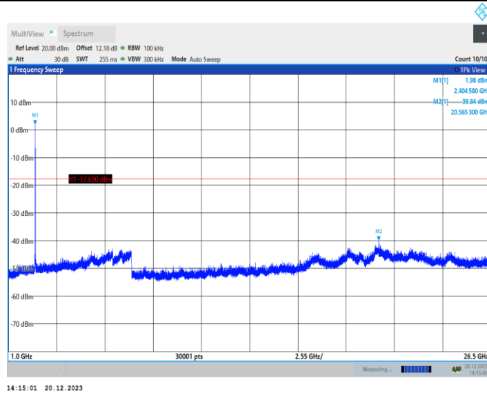
11AX40MIMO_Ant2_2422_106Tone_RU53_0-Reference
