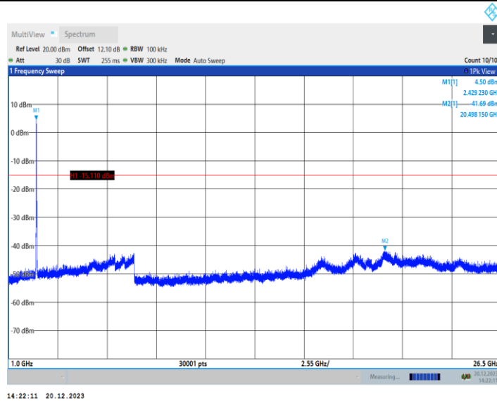
11AX40MIMO_Ant2_2437_26Tone_RU0_0~Reference
