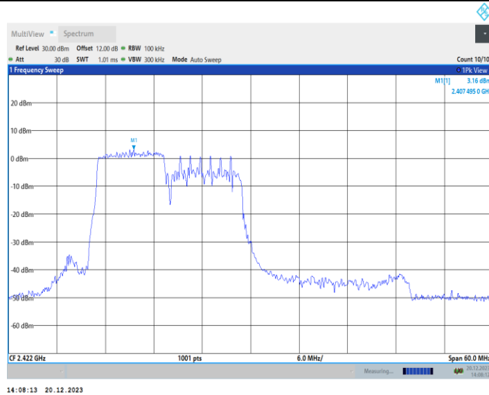
11AX40MIMO_Ant1_2422_106Tone_RU53_30~1000
