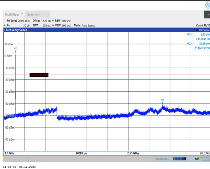
11AX20MIMO_Ant2_2462_106Tone_RU53_0~Reference
