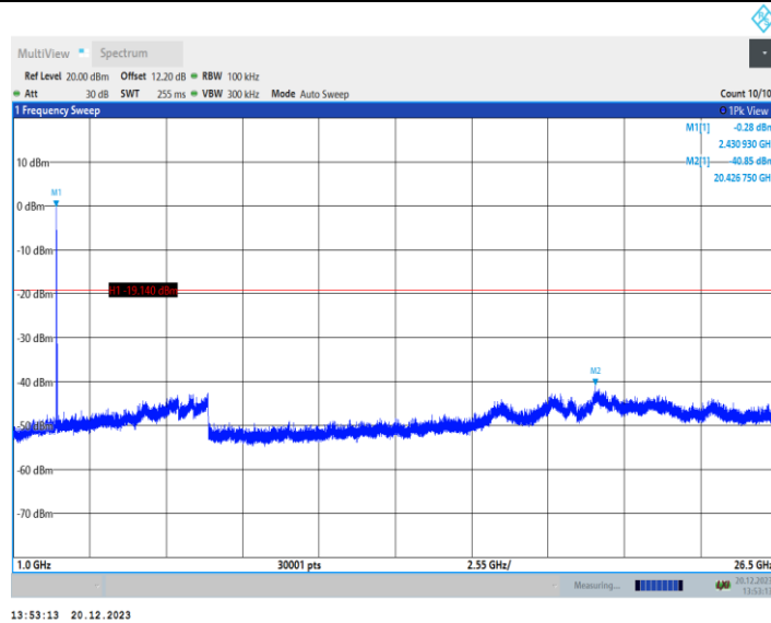
11AX20MIMO_Ant2_2437_106Tone_RU53_0~Reference
