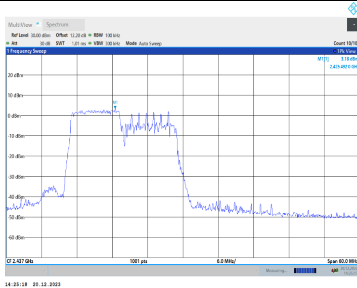
11AX40MIMO_Ant2_2437_106Tone_RU53_30~1000
