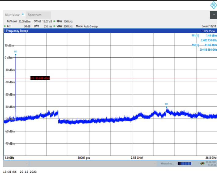
11AX20MIMO_Ant2_2412_26Tone_RU0_0~Reference
