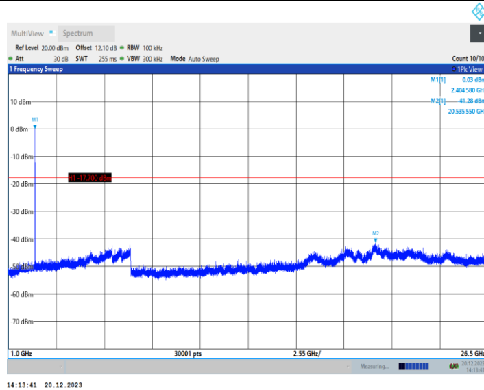
11AX40MIMO_Ant2_2422_52Tone_RU37_0-Reference
