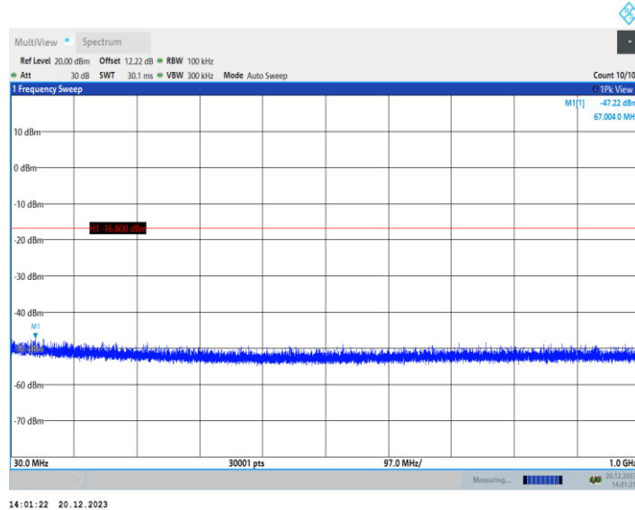
11AX20MIMO_Ant2_2462_26Tone_RU0_1000~26500
