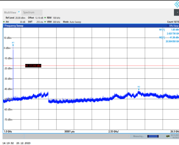
11AX40MIMO_Ant1_2437_106Tone_RU53_0-Reference
