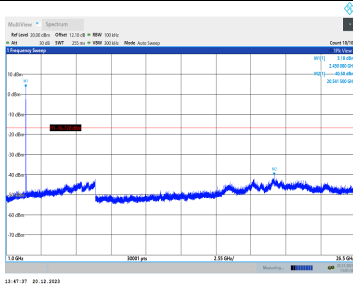
11AX20MIMO_Ant1_2437_106Tone_RU53_0~Reference
