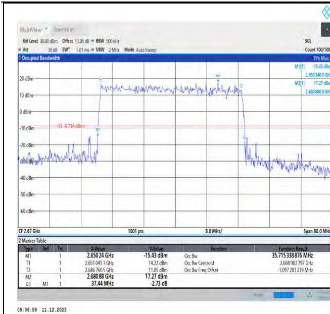
NTNV_N41_PC3_30_40_H_TID1_Ant1#1
