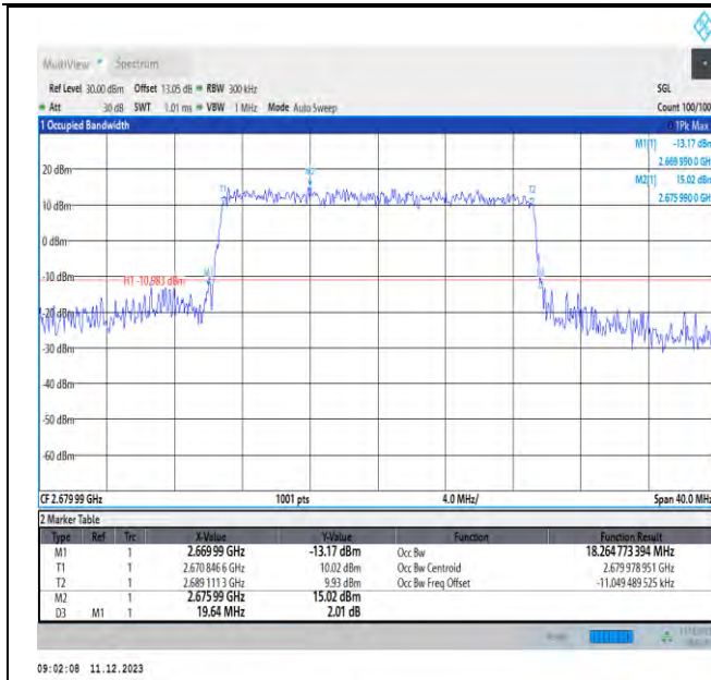
NTNV_N41_PC3_30_20_H_TID5_Ant1#1
