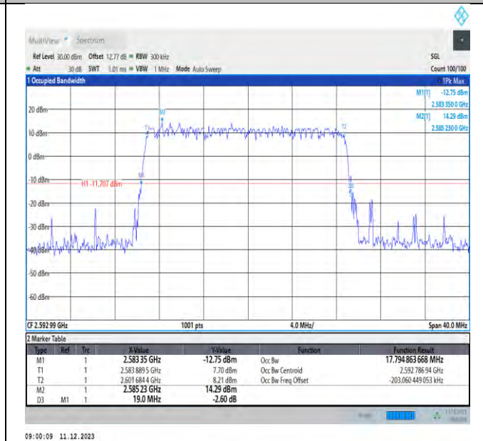
NTNV_N41_PC3_30_20_M_TID4_Ant1#1
