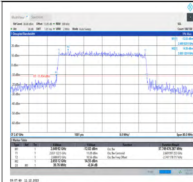
NTV_N41_PC3_30_40_H_TID5_Ant1#1
