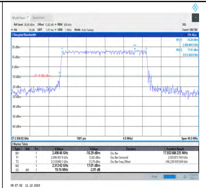
NTNV_N41_PC3_30_20_L_TID2_Ant1#1
