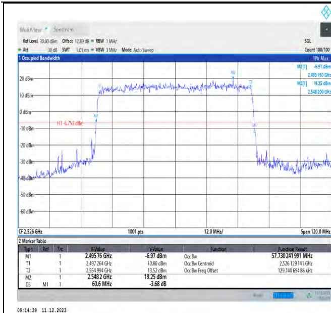
NTNV_N41_PC3_30_60_L_TID1_Ant1#1
