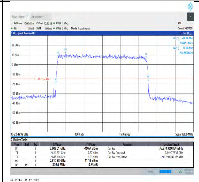
NTNV_N41_PC3_30_80_H_TID8_Ant1#1
