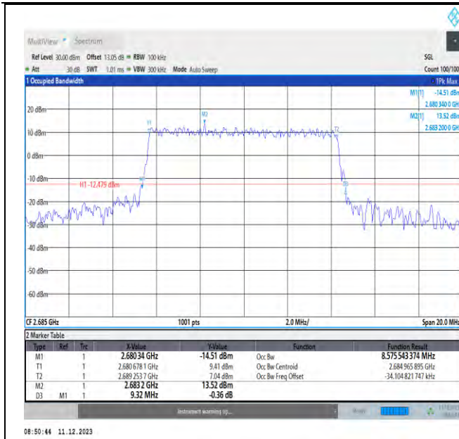
NTNV_N41_PC3_30_10_H_TID5_Ant1#1
