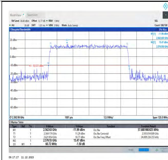
NTNV_N41_PC3_30_60_M_TID5_Ant1#1
