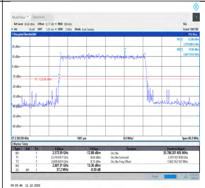
NTNV_N41_PC3_30_40_M_TID4_Ant1#1
