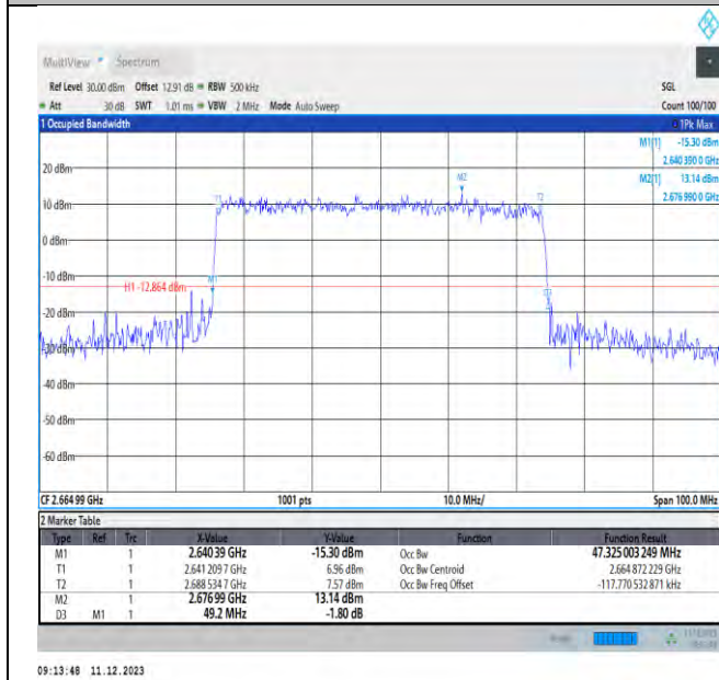
NTNV_N41_PC3_30_50_H_TID7_Ant1#1
