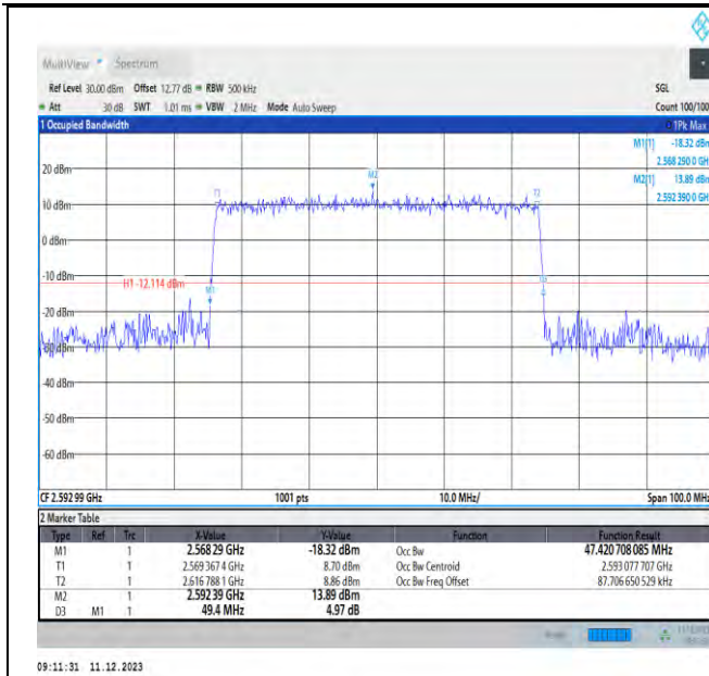
NTNV_N41_PC3_30_50_M_TID5_Ant1#1
