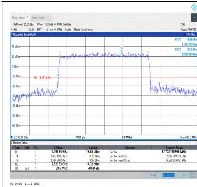
NTNV_N41_PC3_30_40_L_TID5_Ant1#1
