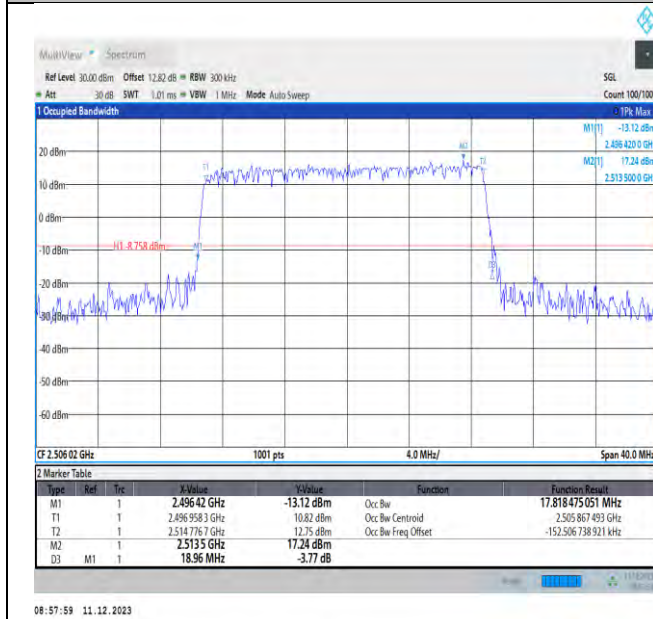
NTNV_N41_PC3_30_20_L_TID3_Ant1#1
