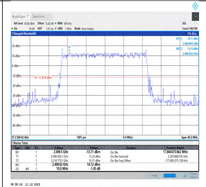
NTNV_N41_PC3_30_20_L_TID4_Ant1#1
