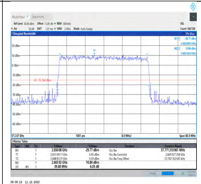
NTV_N41_PC3_30_40_H_TID8_Ant1#1
