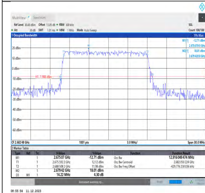
NTNV_N41_PC3_30_15_H_TID3_Ant1#1
