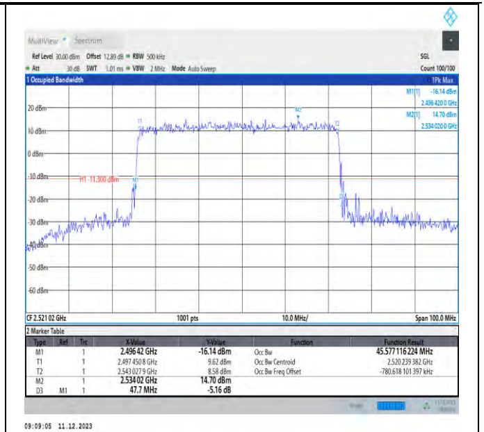
NTNV_N41_PC3_30_50_L_TID2_Ant1#1
