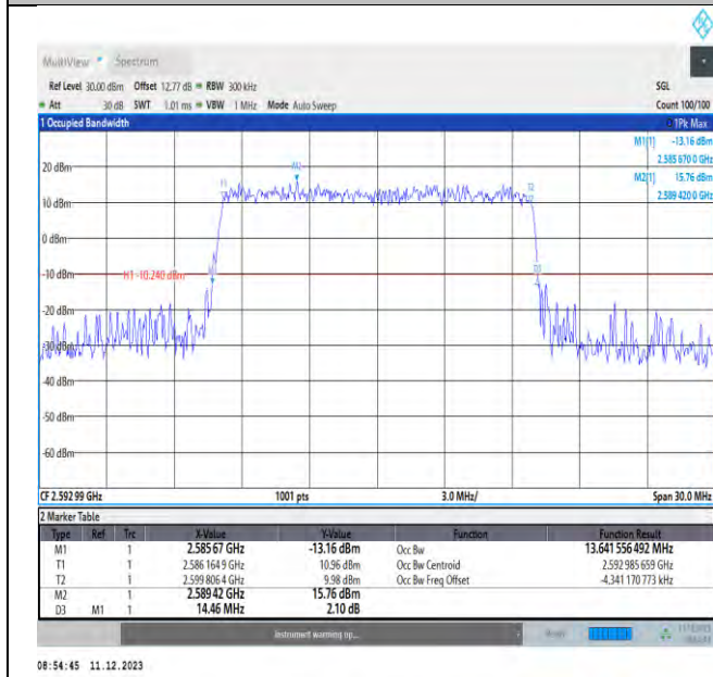
NTNV_N41_PC3_30_15_M_TID7_Ant1#1
