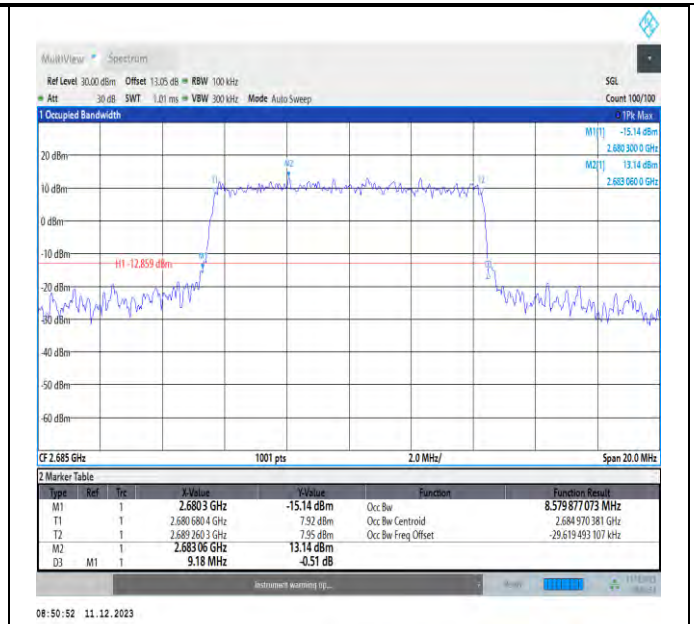
NTNV_N41_PC3_30_10_H_TID6_Ant1#1
