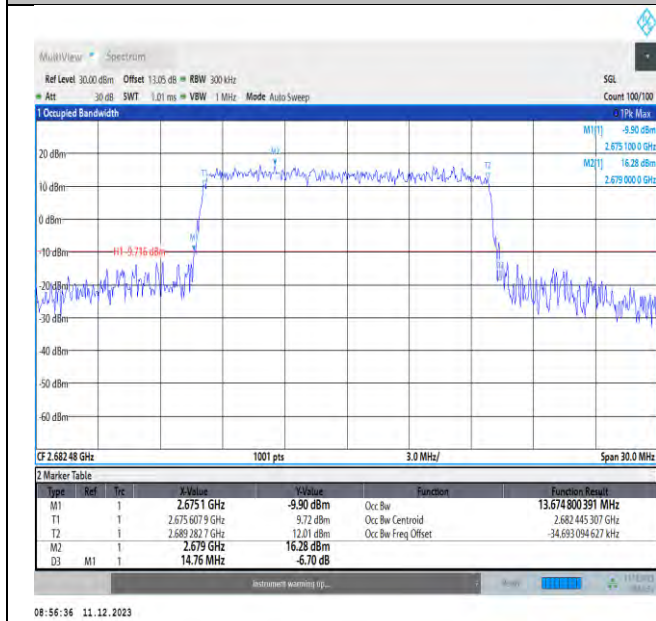
NTNV_N41_PC3_30_15_H_TID7_Ant1#1
