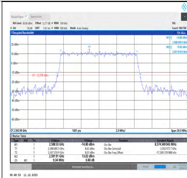
NTNV_N41_PC3_30_10_M_TID5_Ant1#1
