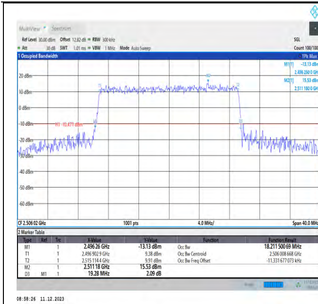
NTNV_N41_PC3_30_20_L_TID5_Ant1#1
