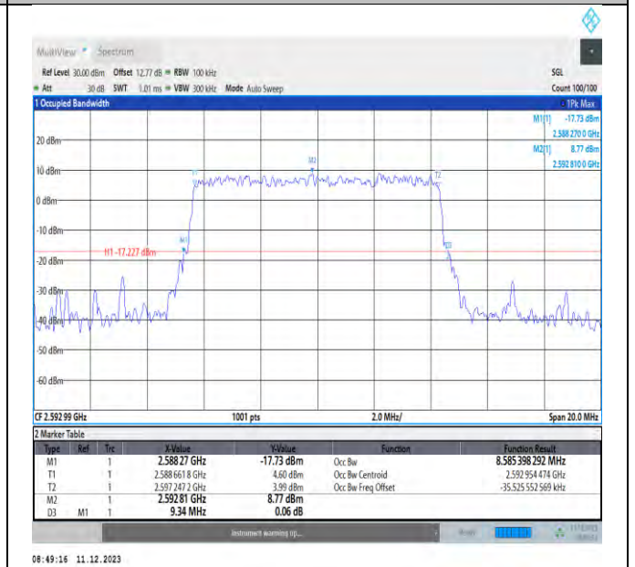
NTNV_N41_PC3_30_10_M_TID8_Ant1#1
