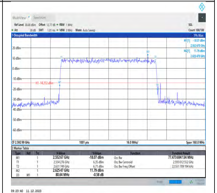
NTNV_N41_PC3_30_80_M_TID8_Ant1#1
