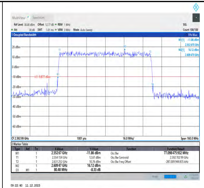
NTNV_N41_PC3_30_80_M_TID2_Ant1#1
