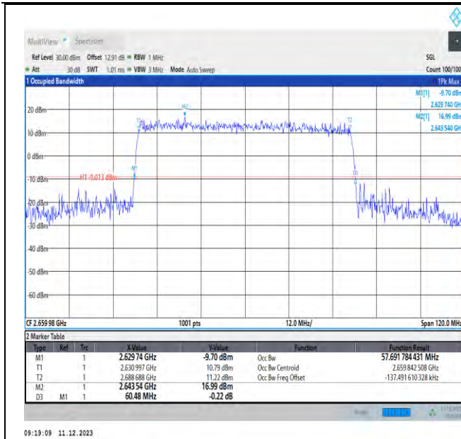
NTV_N41_PC3_30_60_H_TID5_Ant1#1
