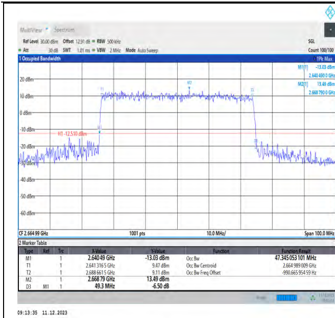
NTNV_N41_PC3_30_50_H_TID5_Ant1#1
