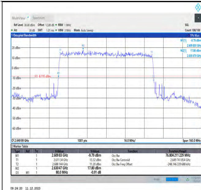
NTNV_N41_PC3_30_80_H_TID1_Ant1#1
