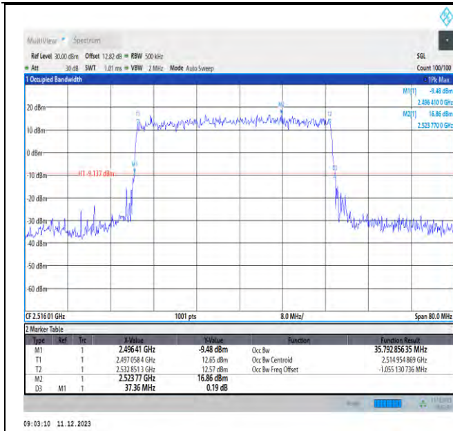
NTNV_N41_PC3_30_40_L_TID1_Ant1#1
