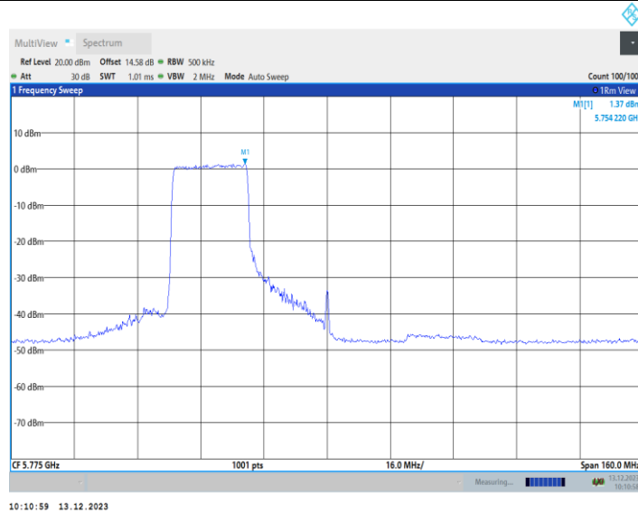
11AX80MIMO_Ant1_5775_484Tone_RU65
