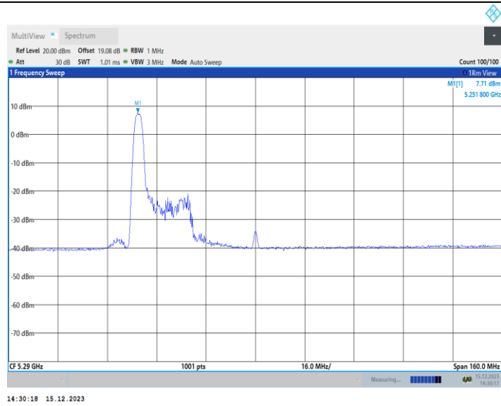
11AX80MIMO_Ant2_5290_52Tone_RU37
