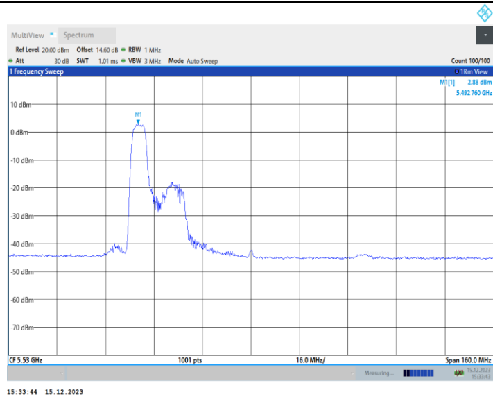
11AX80MIMO_Ant1_5530_106Tone_RU53
