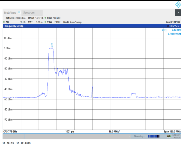
11AX80MIMO_Ant1_5775_106Tone_RU53
