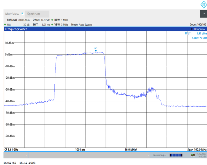
11AX80MIMO_Ant2_5610_26Tone_RU0
