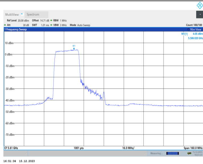
11AX80MIMO_Ant1_5610_484Tone_RU65
