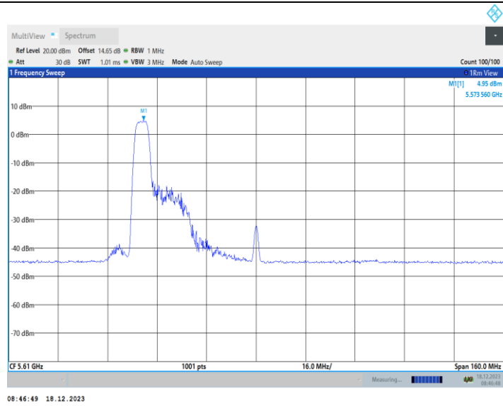
11AX80MIMO_Ant2_5610_106Tone_RU53
