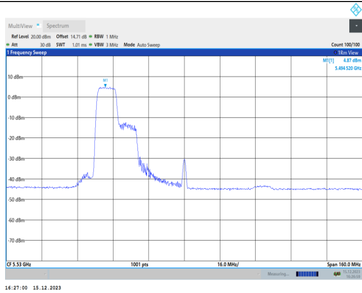
11AX80MIMO_Ant2_5530_242Tone_RU64
