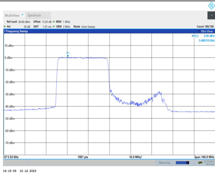
11AX80MIMO_Ant2_5530_26Tone_RU0
