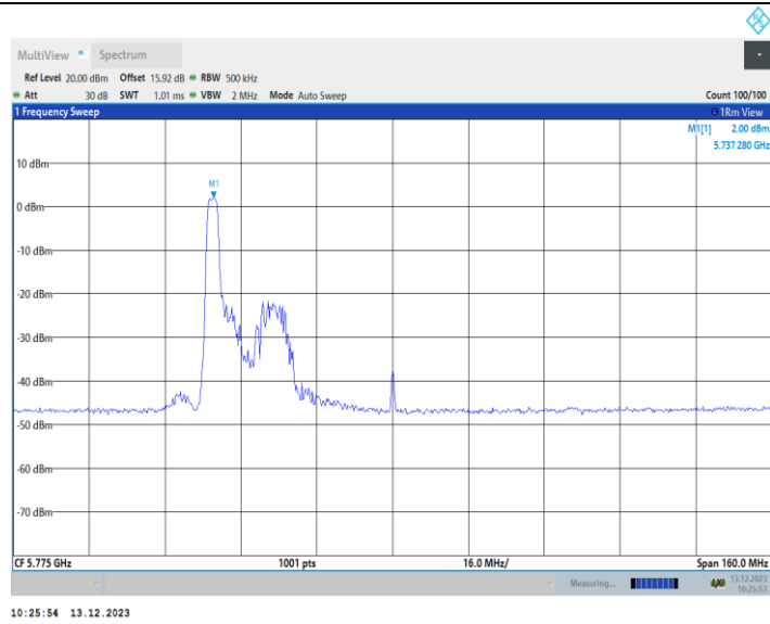
11AX80MIMO_Ant2_5775_52Tone_RU37
