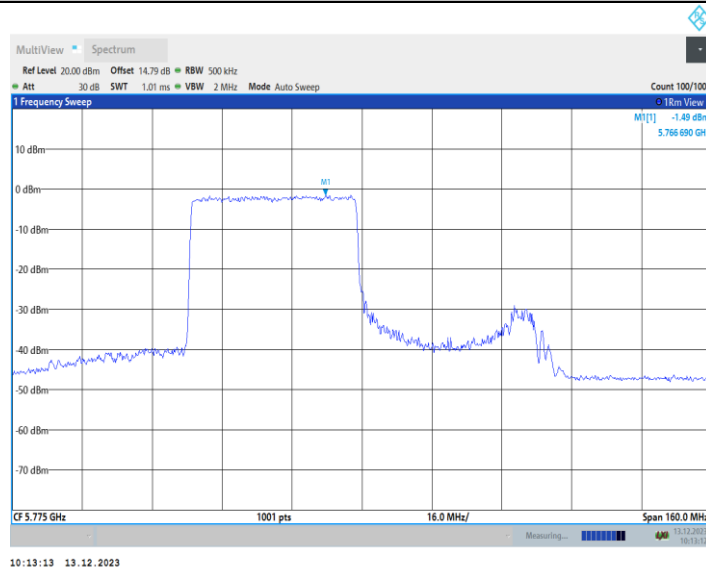
11AX80MIMO_Ant2_5775_26Tone_RU0
