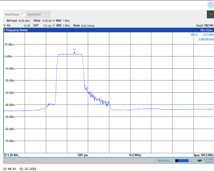
11AX80MIMO_Ant1_5290_484Tone_RU65
