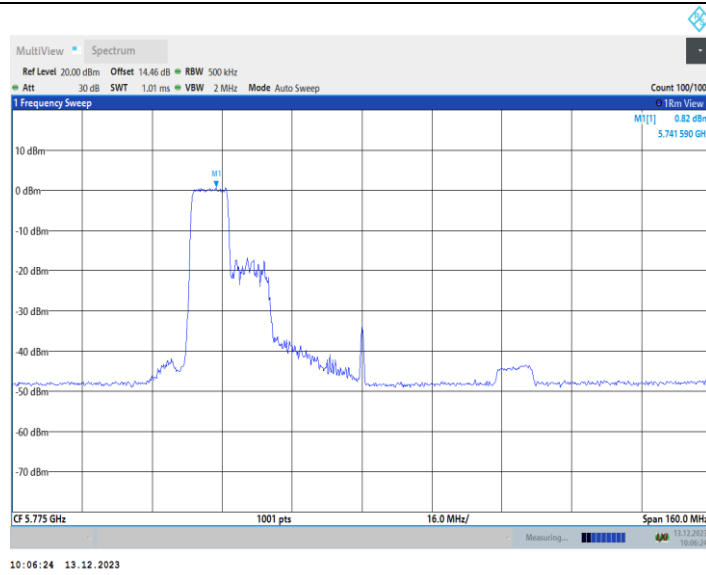
11AX80MIMO_Ant1_5775_242Tone_RU64
