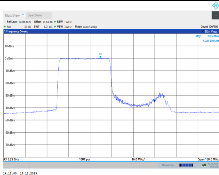
11AX80MIMO_Ant2_5290_26Tone_RU0
