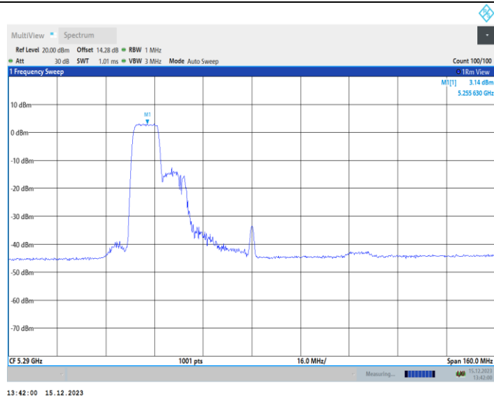
11AX80MIMO_Ant1_5290_242Tone_RU64
