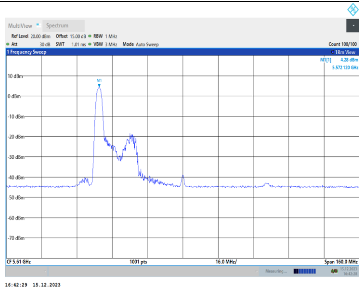
11AX80MIMO_Ant1_5610_52Tone_RU37
