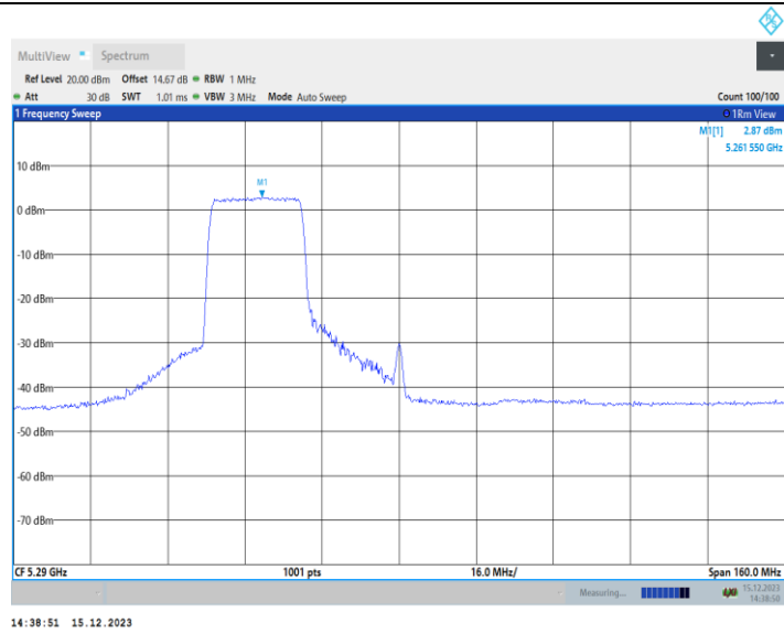
11AX80MIMO_Ant2_5290_484Tone_RU65
