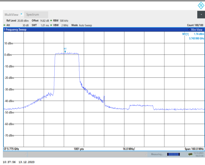
11AX80MIMO_Ant2_5775_484Tone_RU65
