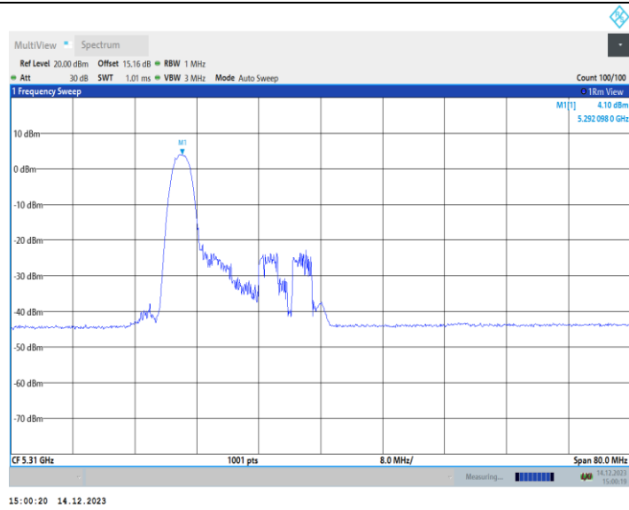
11AX40MIMO_Ant1_5310_52Tone_RU37
