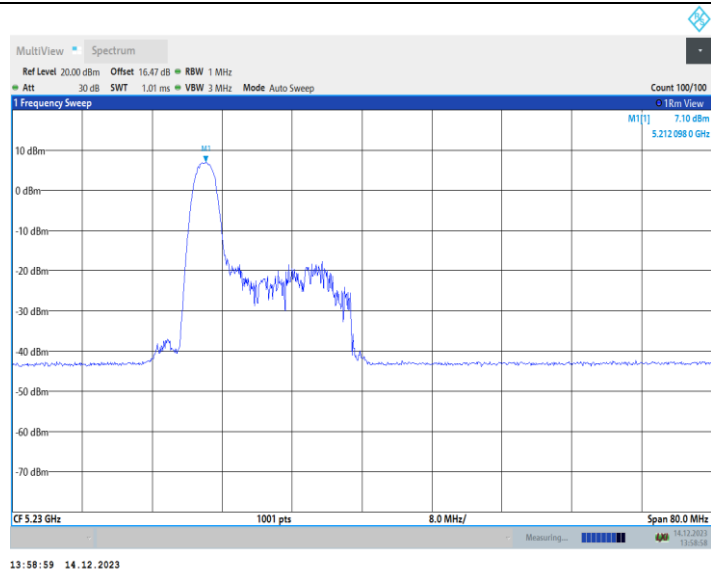
11AX40MIMO_Ant2_5230_52Tone_RU37
