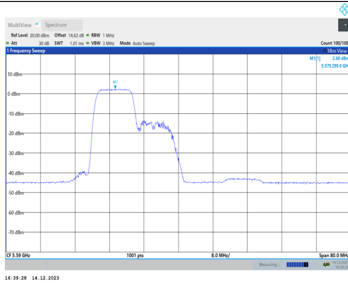
11AX40MIMO_Ant1_5590_242Tone_RU61
