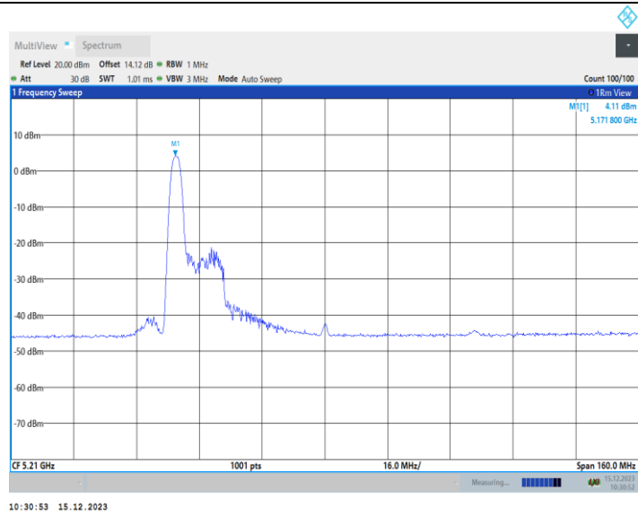
11AX80MIMO_Ant1_5210_52Tone_RU37
