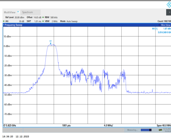
11AX20MIMO_Ant2_5825_52Tone_RU37
