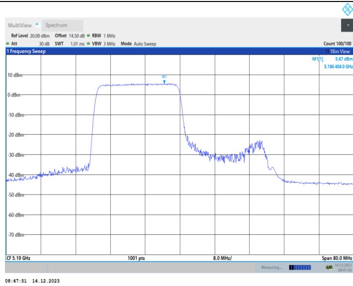
11AX40MIMO_Ant2_5190_26Tone_RU0
