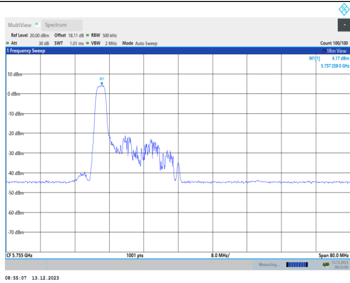
11AX40MIMO_Ant2_5755_52Tone_RU37
