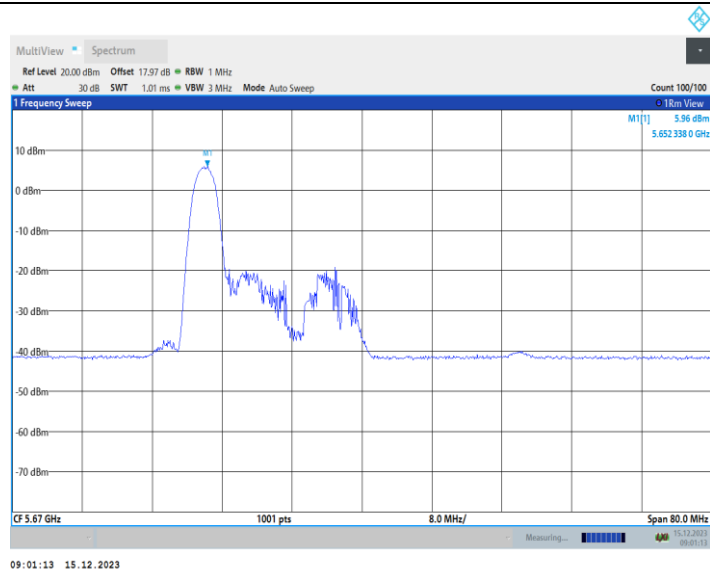
11AX40MIMO_Ant1_5670_52Tone_RU37
