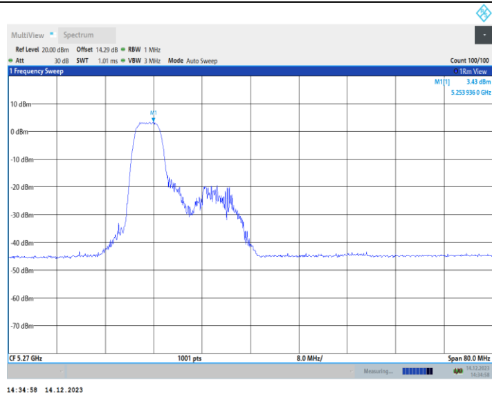
11AX40MIMO_Ant2_5270_106Tone_RU53
