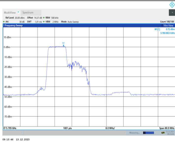
11AX40MIMO_Ant1_5795_242Tone_RU61
