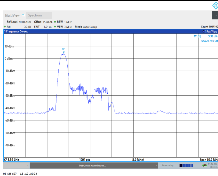
11AX40MIMO_Ant2_5590_52Tone_RU37
