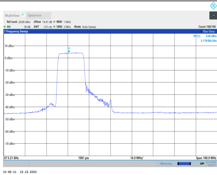
11AX80MIMO_Ant1_5210_484Tone_RU65
