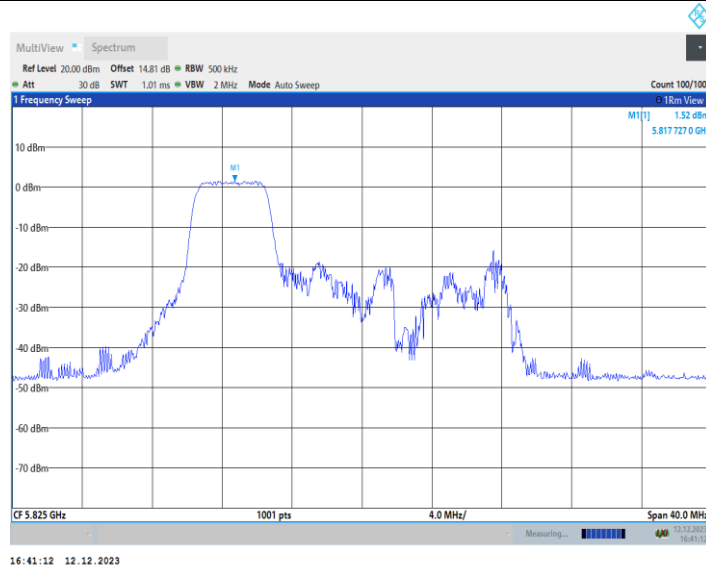
11AX20MIMO_Ant2_5825_106Tone_RU53
