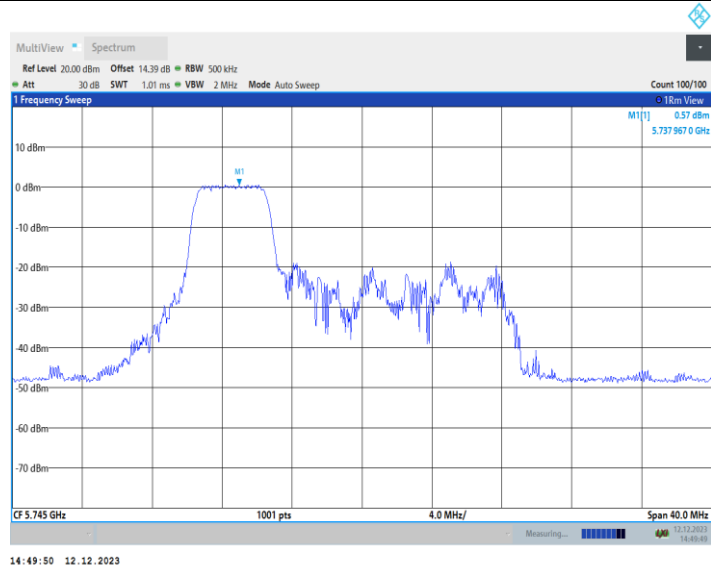
11AX20MIMO_Ant1_5745_106Tone_RU53
