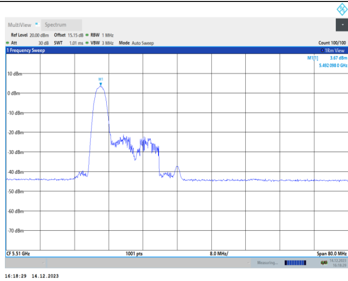
11AX40MIMO_Ant2_5510_52Tone_RU37
