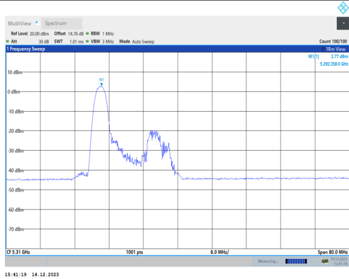
11AX40MIMO_Ant2_5310_52Tone_RU37
