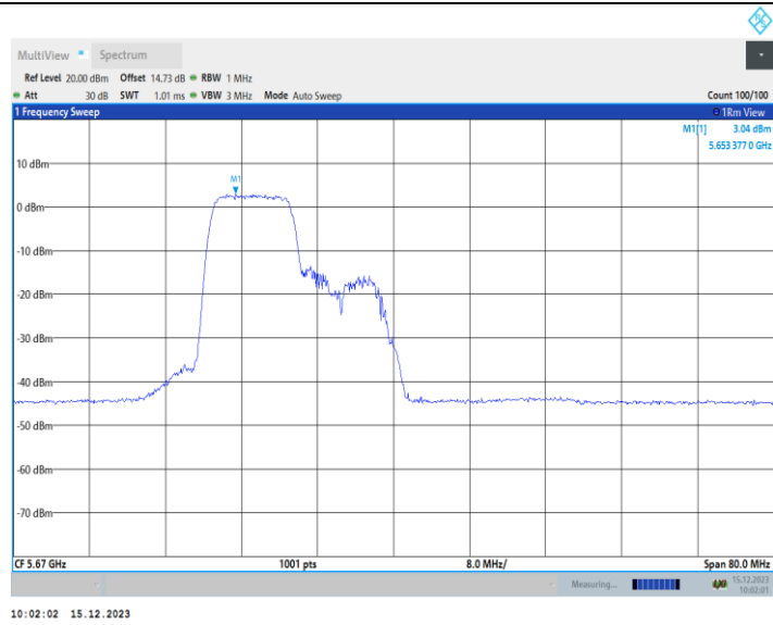
11AX40MIMO_Ant2_5670_242Tone_RU61
