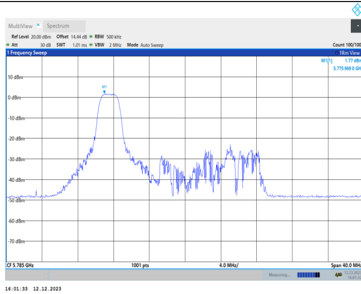
11AX20MIMO_Ant2_5785_52Tone_RU37
