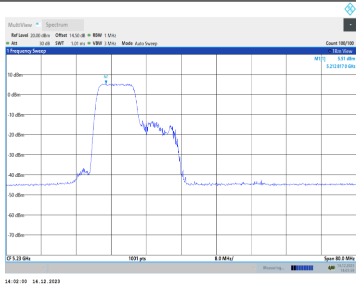
11AX40MIMO_Ant2_5230_242Tone_RU61
