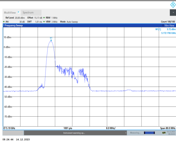
11AX40MIMO_Ant1_5190_52Tone_RU37
