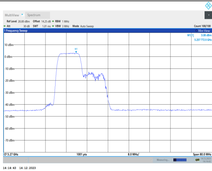
11AX40MIMO_Ant1_5270_242Tone_RU61
