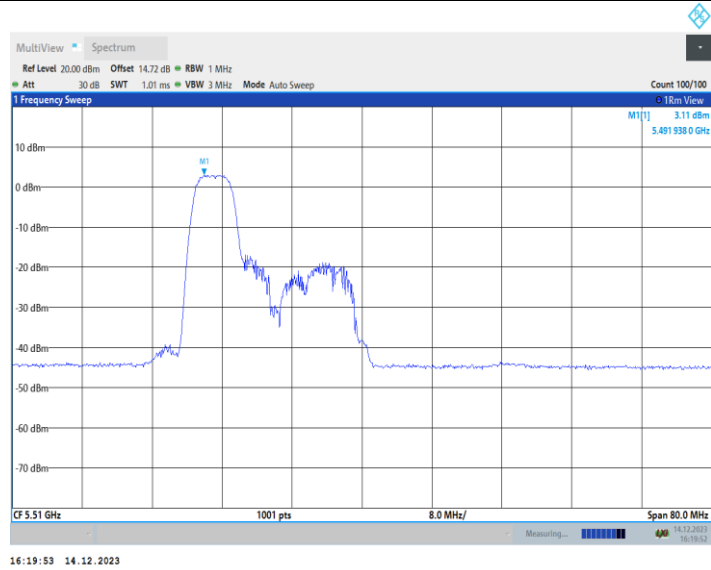
11AX40MIMO_Ant2_5510_106Tone_RU53
