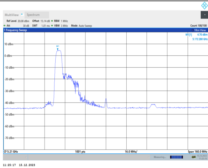
11AX80MIMO_Ant2_5210_106Tone_RU53
