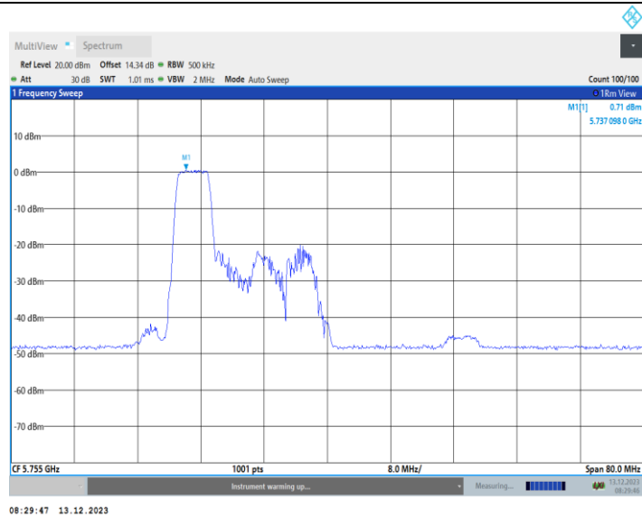
11AX40MIMO_Ant1_5755_106Tone_RU53
