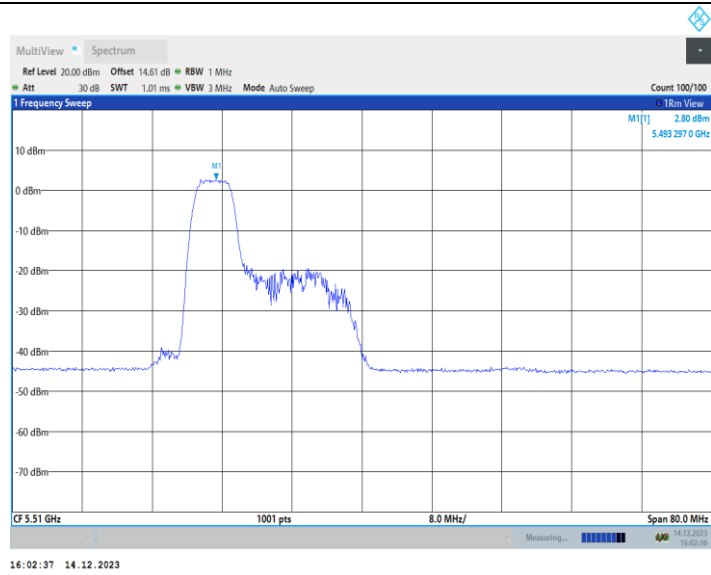
11AX40MIMO_Ant1_5510_106Tone_RU53
