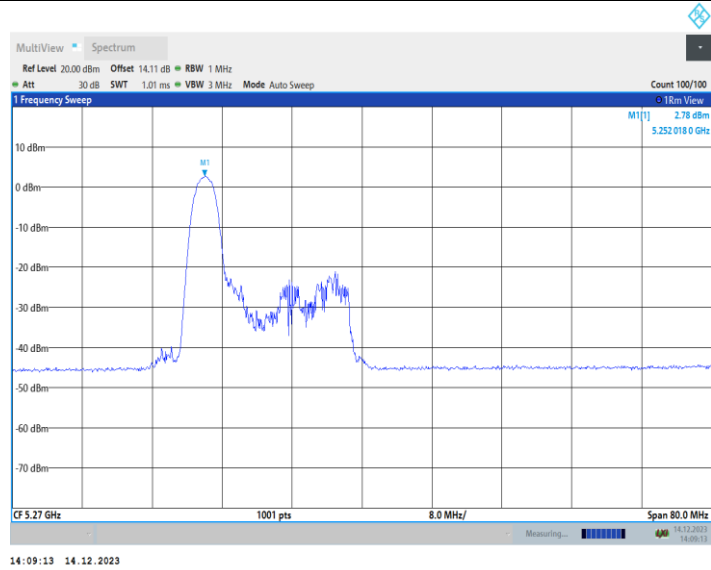
11AX40MIMO_Ant1_5270_52Tone_RU37
