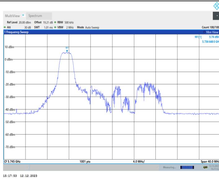
11AX20MIMO_Ant2_5745_52Tone_RU37
