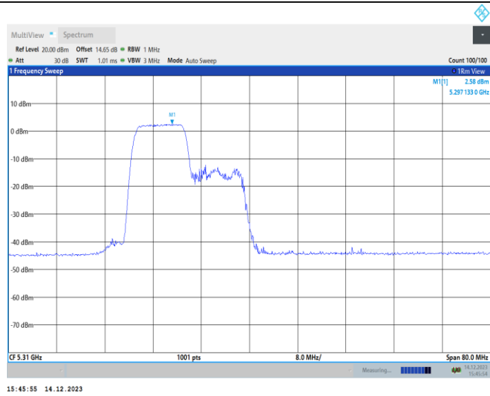
11AX40MIMO_Ant2_5310_242Tone_RU61
