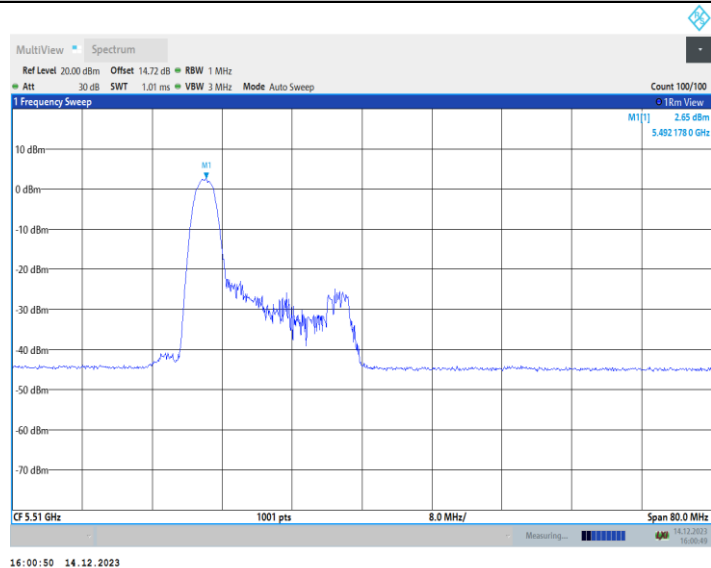
11AX40MIMO_Ant1_5510_52Tone_RU37
