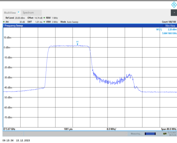
11AX40MIMO_Ant2_5670_26Tone_RU0
