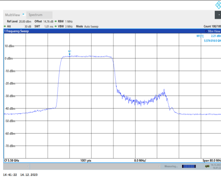
11AX40MIMO_Ant2_5590_26Tone_RU0
