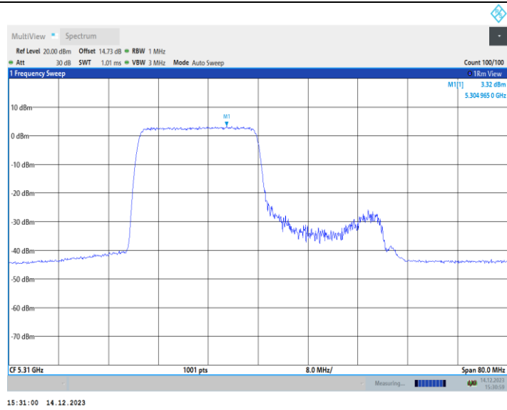
11AX40MIMO_Ant2_5310_26Tone_RU0
