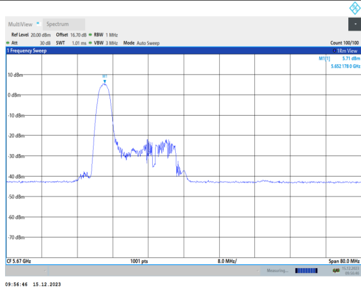
11AX40MIMO_Ant2_5670_52Tone_RU37
