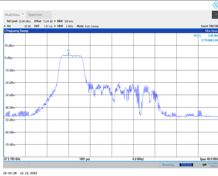
11AX20MIMO_Ant2_5785_106Tone_RU53
