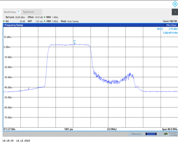
11AX40MIMO_Ant2_5270_26Tone_RU0
