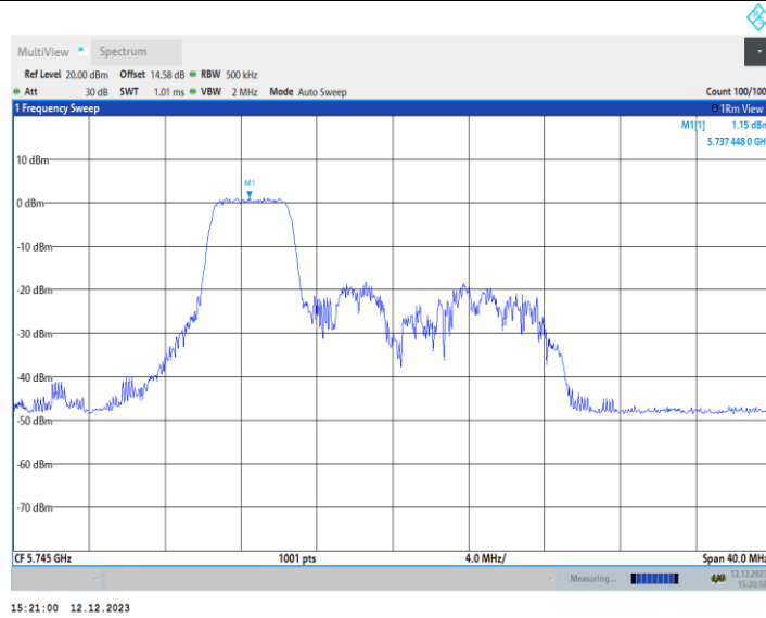
11AX20MIMO_Ant2_5745_106Tone_RU53
