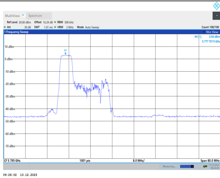
11AX40MIMO_Ant2_5795_106Tone_RU53
