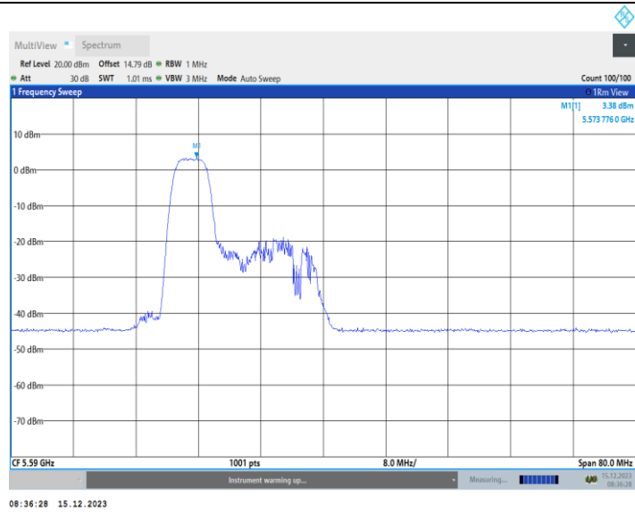
11AX40MIMO_Ant2_5590_106Tone_RU53
