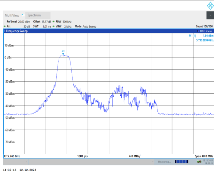
11AX20MIMO_Ant1_5745_52Tone_RU37
