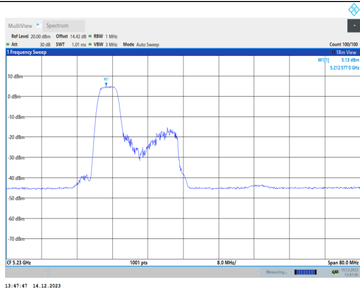
11AX40MIMO_Ant1_5230_106Tone_RU53
