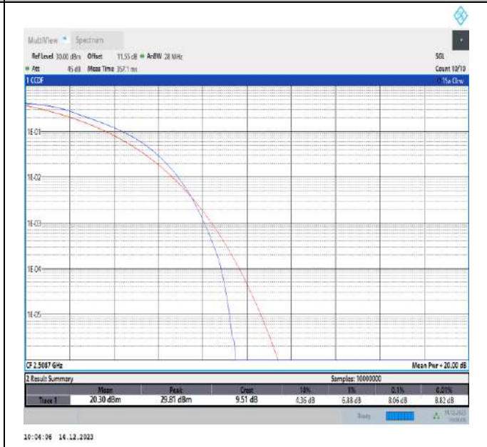
41-41-10MHz-20MHz-QPSK-QPSK-39705-39849-50RB#0-100RB#0-PASS
