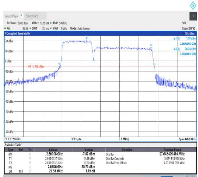
41-41-10MHz-20MHz-QPSK-QPSK-39705-39849-50RB#0-100RB#0-PASS
