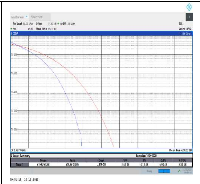
7-7-20MHz-10MHz-QPSK-QPSK-21051-21195-100RB#0-50RB#0-PASS
