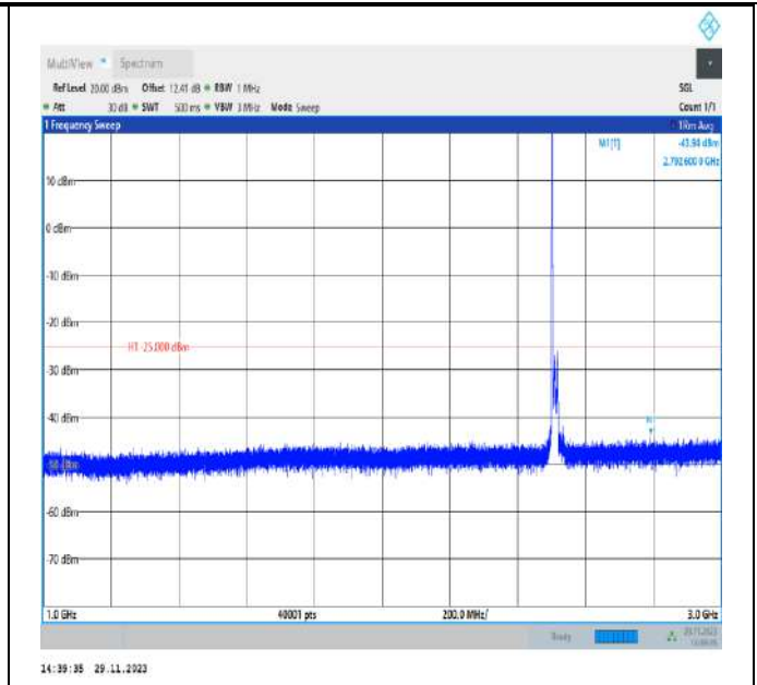
Band7_20MHz_QPSK_20850_1RB#0_1000~3000_1000~3000 00
