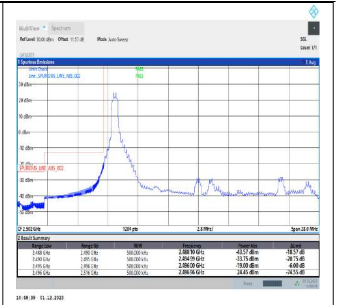
Band41_20MHz_QPSK_39750_1RB#0
