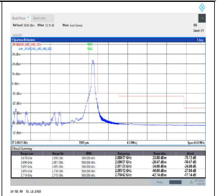
Band41_20MHz_QPSK_41490_1RB#99
