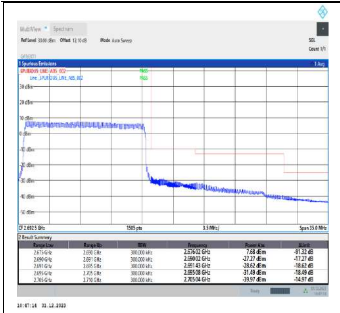
Band41_15MHz_QPSK_41515_75RB#0
