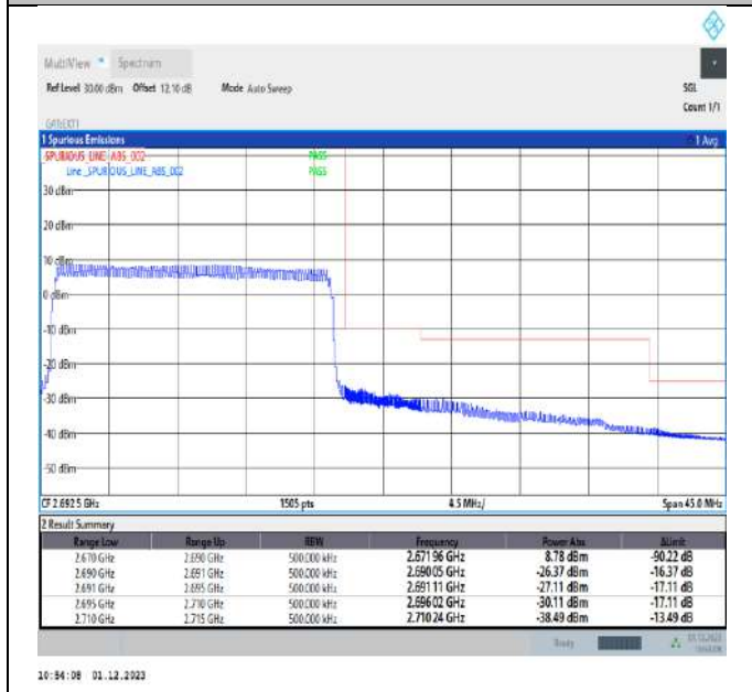
Band41_20MHz_QPSK_41490_100RB#0
