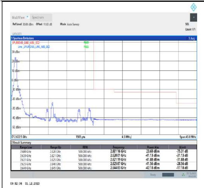
Band38_20MHz_QPSK_38150_1RB#0
