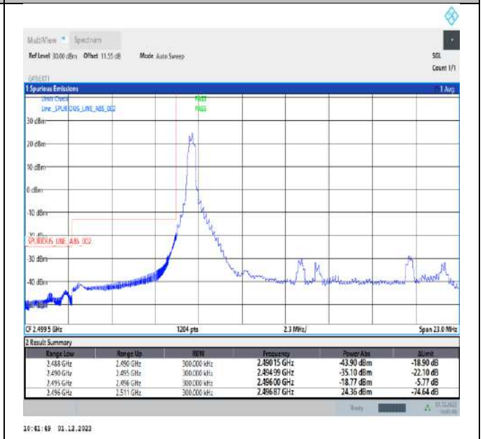
Band41_15MHz_QPSK_39725_1RB#0
