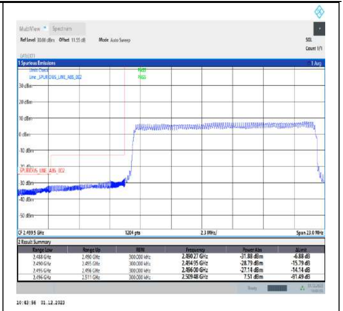
Band41_15MHz_QPSK_39725_75RB#0
