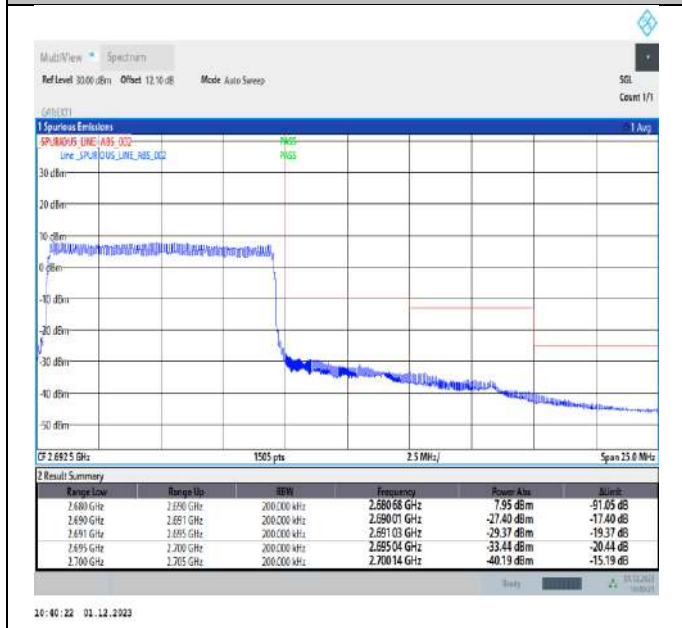
Band41_10MHz_QPSK_41540_50RB#0
