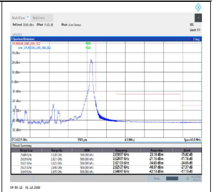
Band38_20MHz_QPSK_38150_1RB#99
