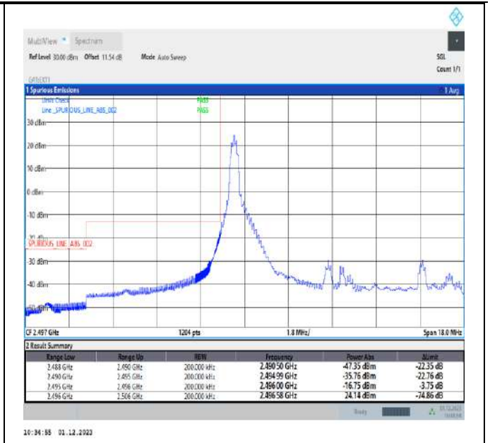
Band41_10MHz_QPSK_39700_1RB#0
