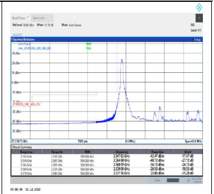
Band38_20MHz_QPSK_37850_1RB#0
