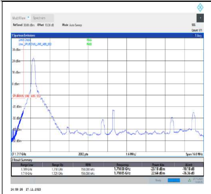
Band4_15MHz_QPSK_2025_1RB#0
