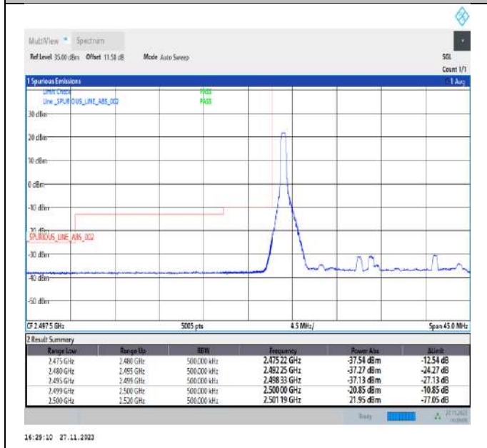
Band7_20MHz_64QAM_20850_1RB#0
