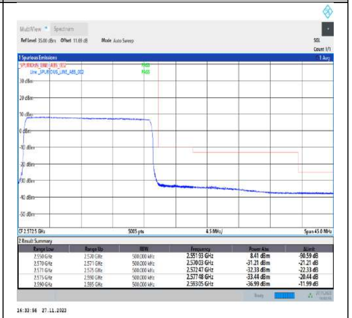
Band7_20MHz_QPSK_21350_100RB#0
