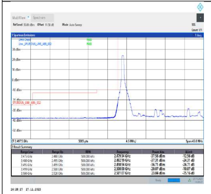
Band7_20MHz_QPSK_20850_1RB#0
