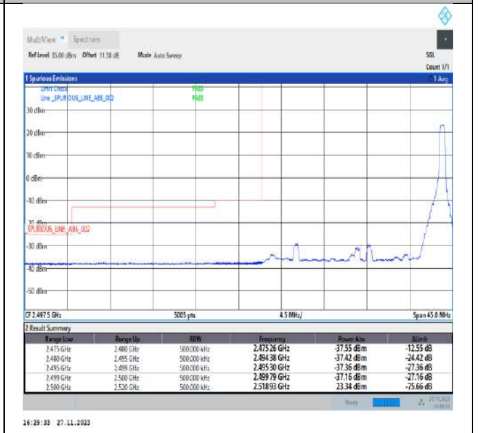
Band7_20MHz_QPSK_20850_1RB#99
